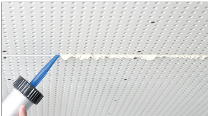
Obr. 4-24 Úplné vyplnění spáry po celé tloušťce desky 20 mm
