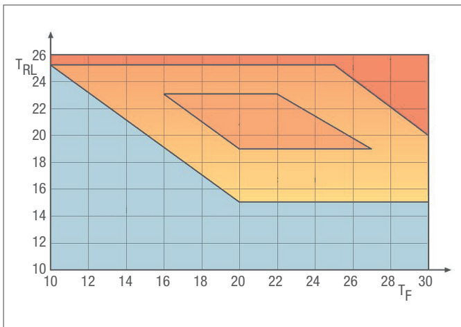
Obr. 2-1 Příjemné teplotní klima, závislé na teplotě vzduchu v místnosti T_{RL} a teplotě ploch obklopujících místnost T_F
