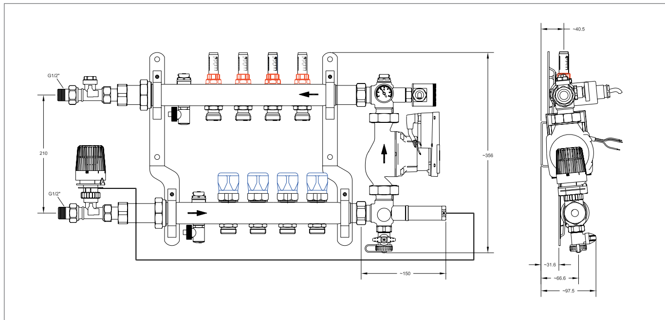
Obr. 10-5 Mísicí sada s HKV-D
