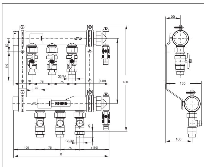
Obr. 17-4 Rozměry
