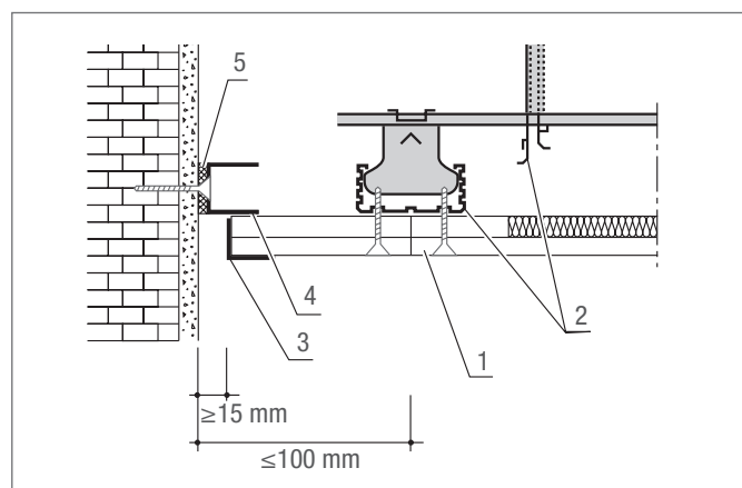
Obr. 5-9 Kluzné napojení na stěnu
