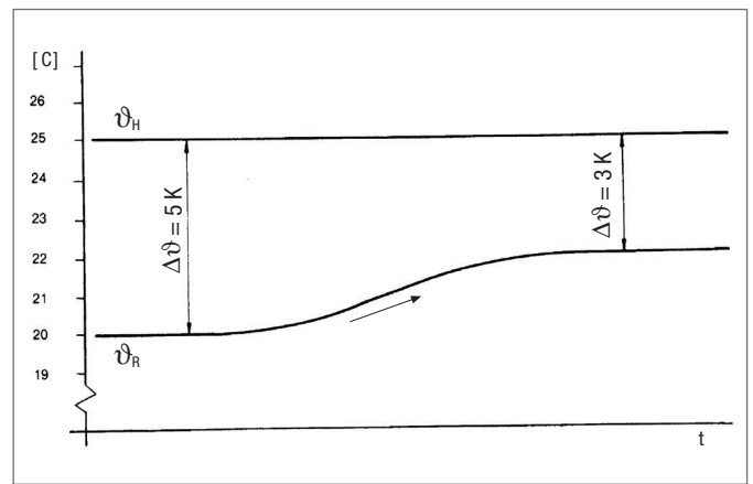
Obr. 10-1 Zobrazení efektu samoregulace:
