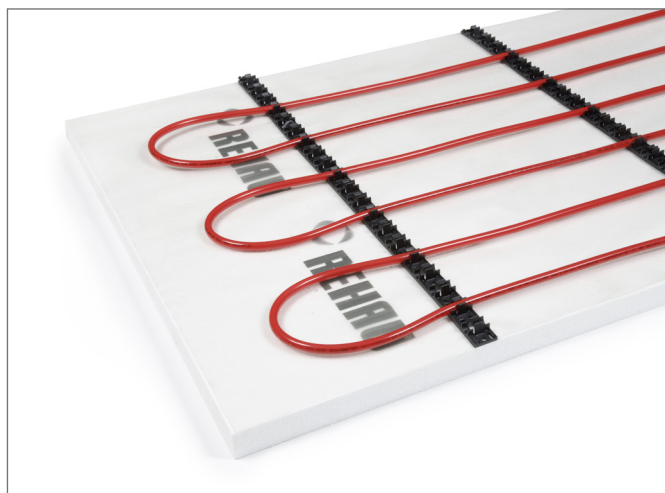
Vodící lišta Raufix
