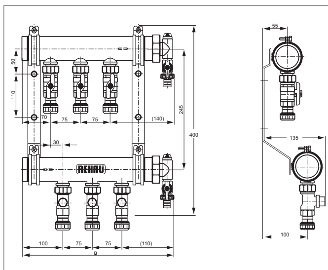
Obr. 17-6 Rozměry
