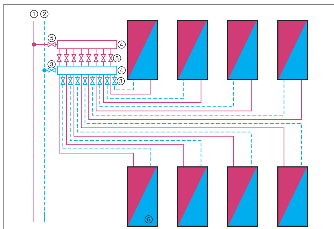
Obr. 11-8 Schématické zobrazení připojení rozdělovače
