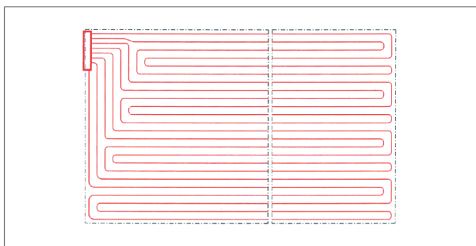
Obr. 12-14 Oddělené topné okruhy
