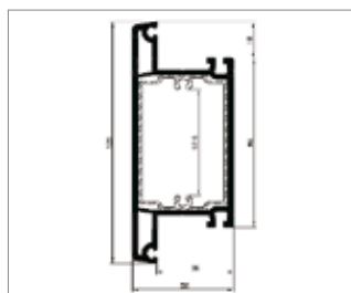
Travessa de folha 120
