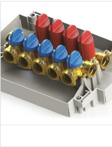
Колектор SMART RAUTITAN LX link
