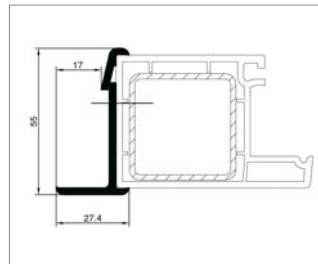
Stulpprofil
