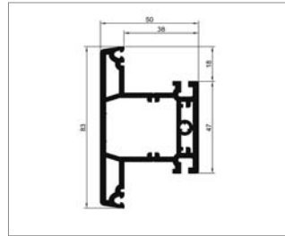
Sprosse 83
