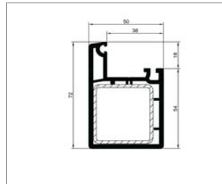
Flügel 72
