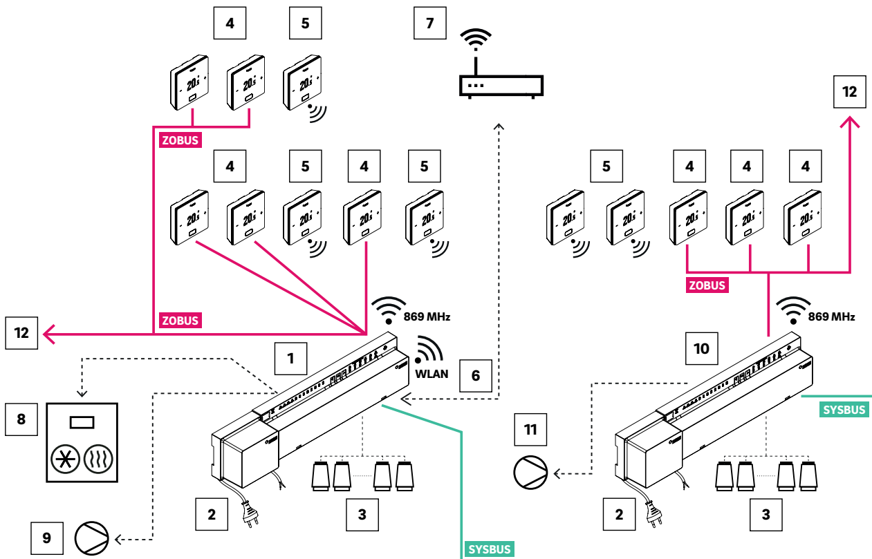
Fig. 02-24 Sistema NEA SMART 2.0, regulación de la temperatura ambiente para calefacción/el refrigeración de hasta 24 recintos mediante el ejemplo de la variante de 24 V
