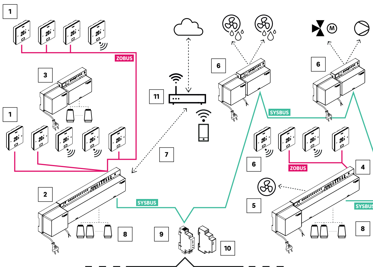
Fig. 02-2 Vista general del sistema NEA SMART 2.0 para 24 V
