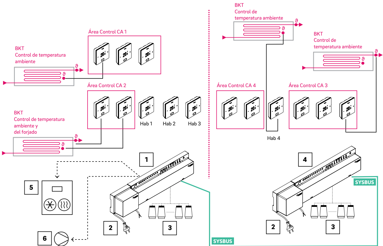
Fig. 02-25 Sistema NEA SMART 2.0, monitorización y zonas de regulación BKT con una unidad esclava (4 zonas de regulación y, adicionalmente, 4 recintos)
