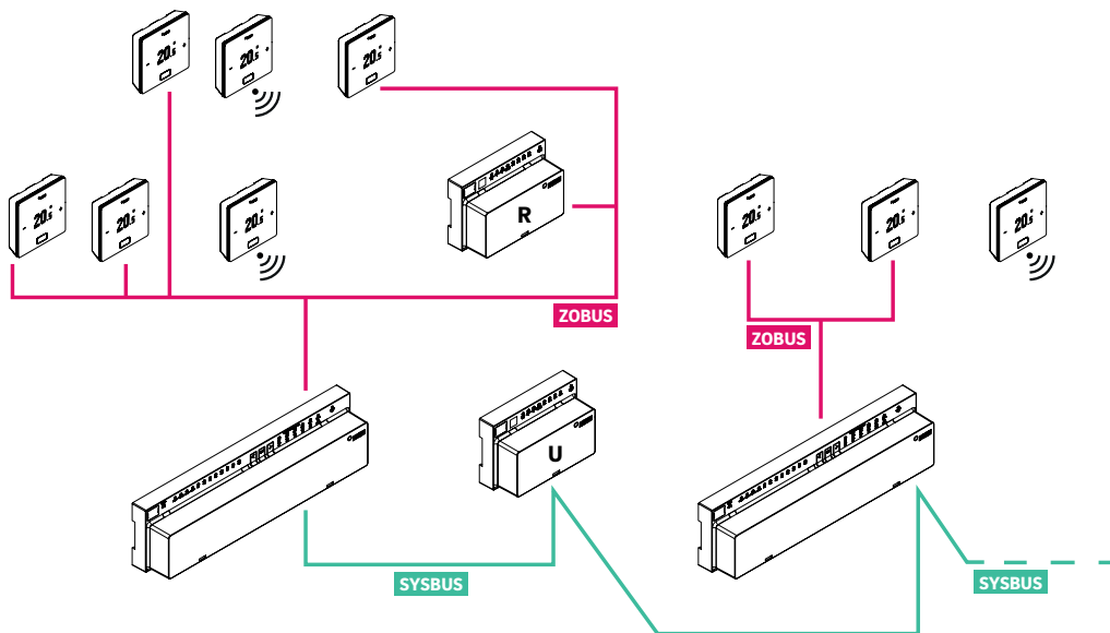
Fig. 02-21 Zone Bus (ZOBUS) y bus de sistema (SYSBUS)
