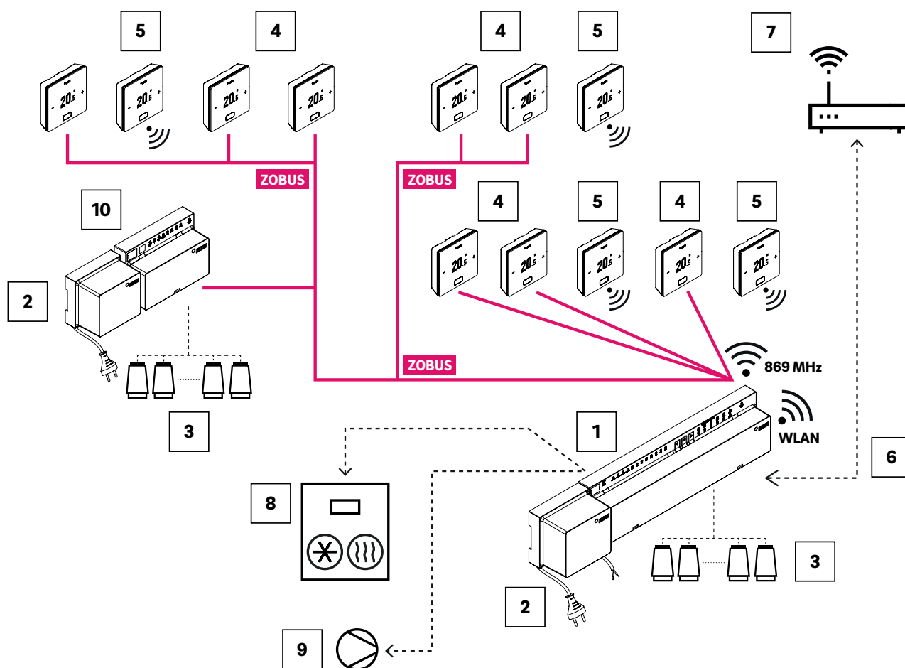
Fig. 02-23 Sistema NEA SMART 2.0, regulación de la temperatura ambiente para calefacción / refrigeración hasta 12 recintos mediante el ejemplo de la variante de 24 V
