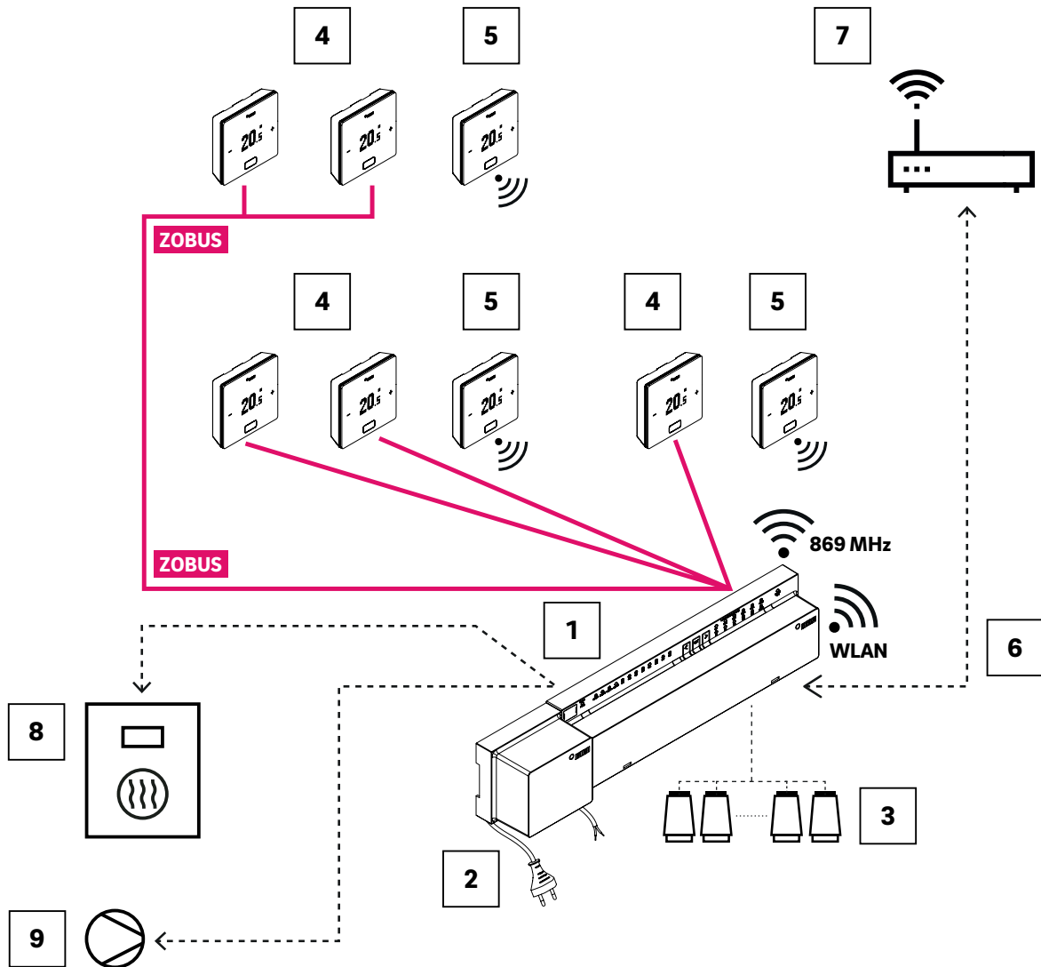
Fig. 02-22 Sistema NEA SMART 2.0, regulación de la temperatura ambiente para calefacción mediante el ejemplo de la variante de 24 V
