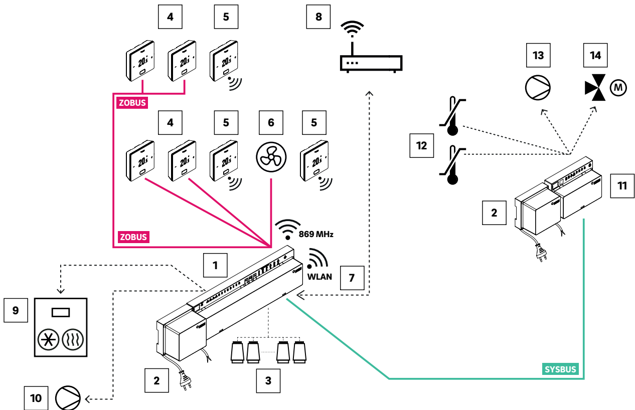
Fig. 02-26 Sistema NEA SMART 2.0, regulación termostática para calefacción/refrigeración con regulación de un circuito de mezcla mediante el ejemplo de la versión de 24 V
