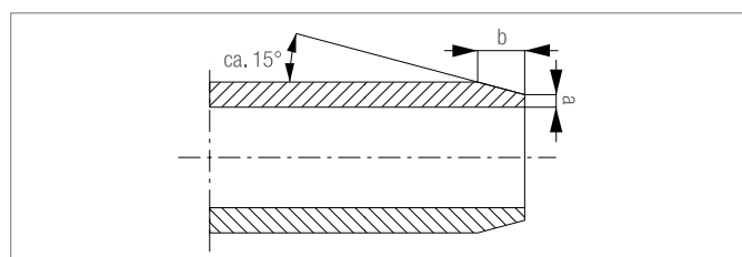
Abb. 4-3 Afschuinen van afgezaagde buisuiteinden
