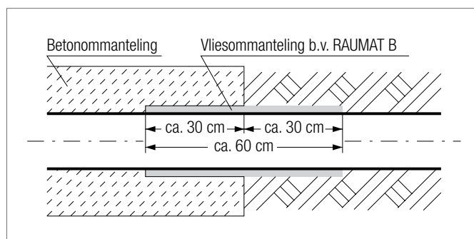
Afb. 5-33 Betonmantel in stromingsrichting van de lucht
