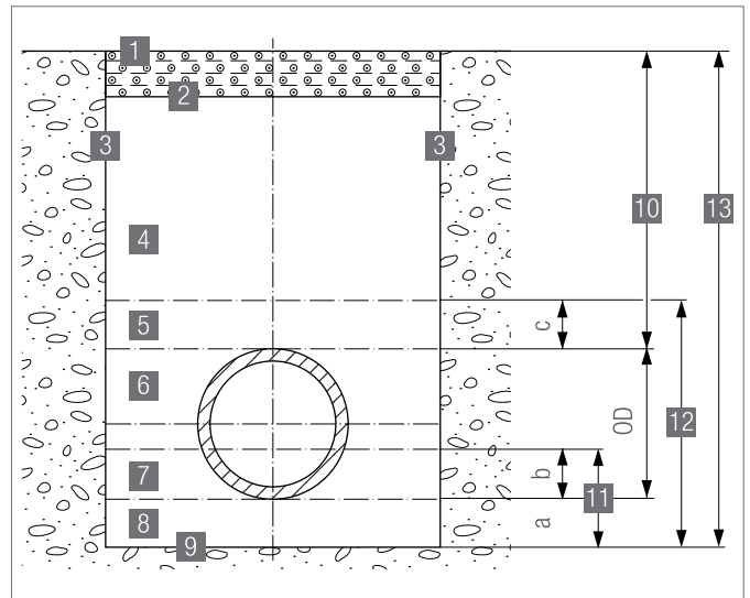
Abb. 4-2 Installeren
