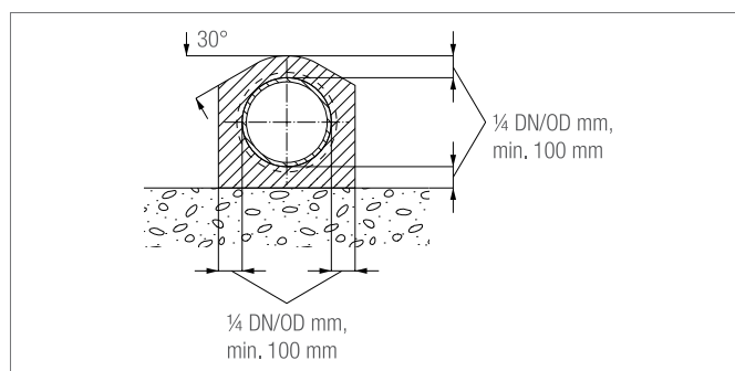
Afb. 5-32 Betonmantel doorsnede
