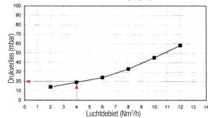
Extra drukverlies door beluchter met terugslagklep
