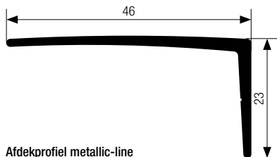
Afdekprofiel metallic-line
