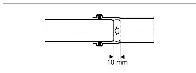
Rys. 5-1 Wykonywanie szczelin dylatacyjnych przez wysunięcie końców rur
