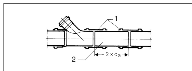
Rys. 5-3 Montaż kształtek
