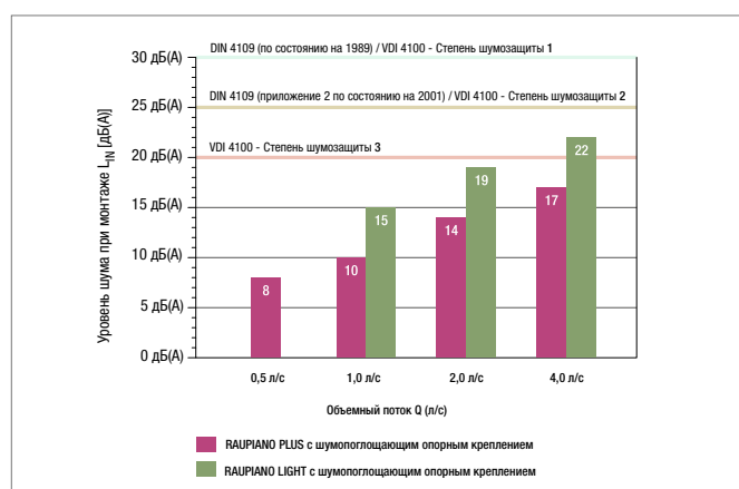
Рис. 5-6 Результаты измерений с использованием шумопоглощающего опорного крепления на нижнем этаже за установочной стеной (источник: Фраунгофский Институт строительной физики, Штутгарт, акт о проведении испытаний P-BA 6/2006)
