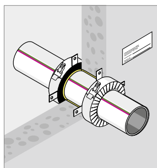
Рис. 6-3 Противопожарная манжета для накладки на вертикальную стену
