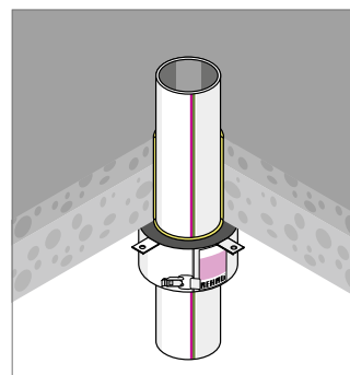
Рис. 6-2 Противопожарная манжета для накладки на перекрытие
