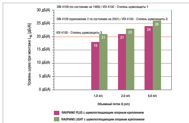
Рис. 5-7 Результаты измерений с использованием стандартного хомута на нижнем этаже за установочной стеной (источник: Фраунгофский Институт строительной физики, Штутгарт, акт о проведении испытаний P-BA 176/2006)
