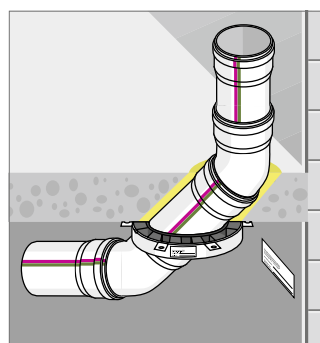
Рис. 6-4 Угловая противопожарная манжета (только для накладки на перекрытие)
