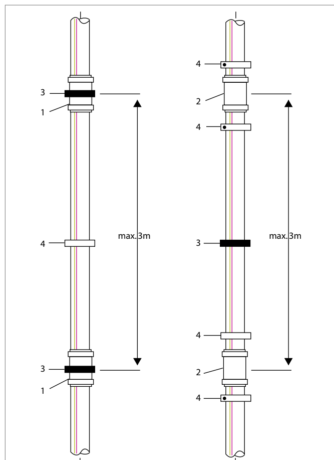
Рис. 8-2 Использование двухраструбных или подвижных муфт
