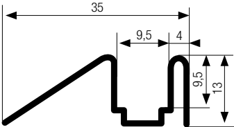
Riel-guía TOP BASIC de 8 mm
