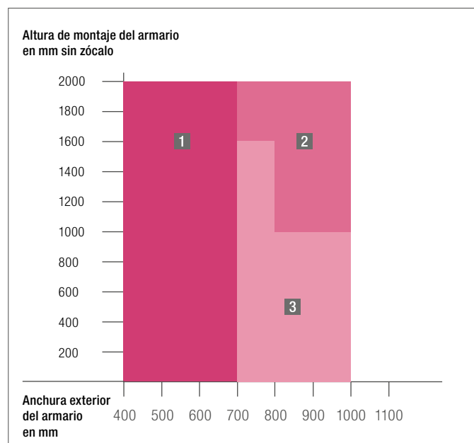
Nº artículo 1793310XXX Mecanismo C8
