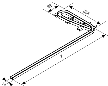
Caracolas-guía izquierda y derecha : x = 400 / 500 / 600 mm Capacidad 600 mm
