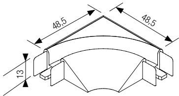
Esquina 90° TOP BASIC 8 mm
