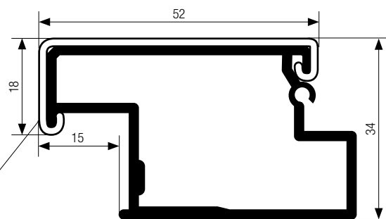
Tirador solapado (embellecedor) color-line / decor-line Tirador (parte inferior) color-line / decor-line (aluminio)
