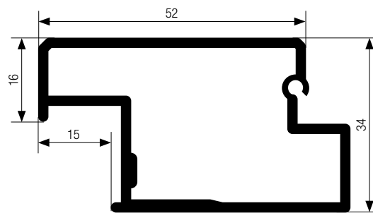
Tirador metallic-line (aluminio / acero inoxidable)
