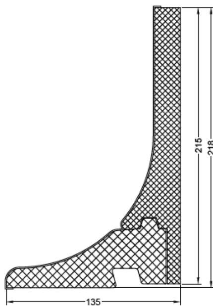
Wärmedämmkeil EG 245 zweiteilig (1,25 m) 287785 ■ 12
