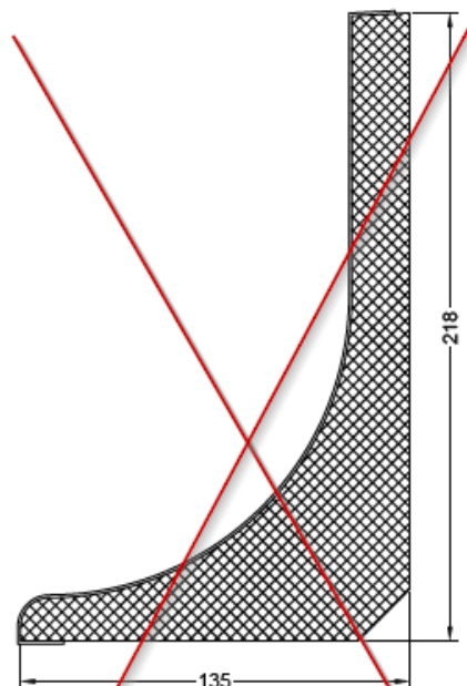
Wärmedämmkeil EG 245 (1,25 m) 287795 ■ 10
