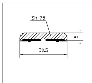
Лента-целик Номер материала: 1712002 Материал: RAU-ПВХ 7589/9808
