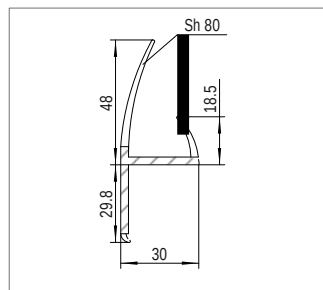
Профиль для уплотнения двери Номер материала: 1601487 Материал: RAU-ПВХ 1309/8058
