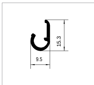
Профиль для защиты кантов
