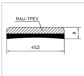
Противоударный защитный профиль Номер материала: 1638013 Материал: RAU-ПП 1381 RAU-TPEV 504
