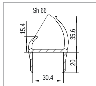
Профиль для уплотнения двери Номер материала: 1600653 (Z) Материал: RAU-ПВХ 1309/6658
