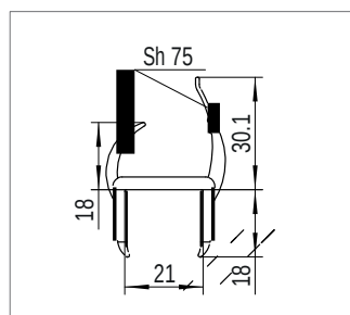
Профиль для уплотнения двери Номер материала: 1610672 Материал: RAU-ПВХ 1309/7558
