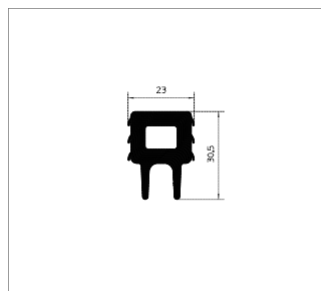
Уплотнительный профиль
