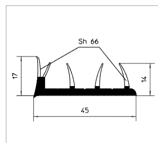
Профиль для уплотнения двери Номер материала: 1635372 Материал: RAU-ПВХ 1103/6658
