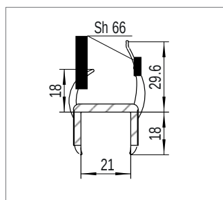
Профиль для уплотнения двери Номер материала: 1600842 Материал: RAU-ПВХ 1309/6658
