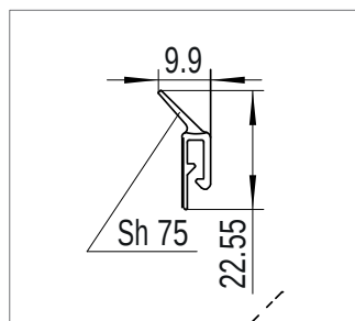
Обшивочный профиль
