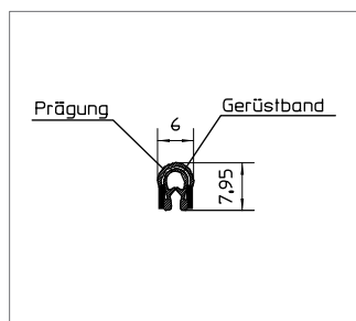
Профиль для защиты кромок армированный металлом Номер материала: 1618304 Материал: RAU-ПВХ 8505
