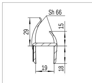
Профиль для уплотнения двери Номер материала: 1636612 (Z) Материал: RAU-ПВХ 1309/6658
