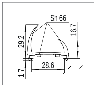
Профиль для уплотнения двери Номер материала: 1633743 (Z) Материал: RAU-ПВХ 1103/6658
