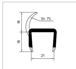
Профиль для уплотнения двери Номер материала: 1610682 Материал: RAU-ПВХ 1309/7558
