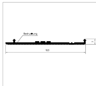
Специальный профиль Номер материала: 1606953 Материал: RAU-ПВХ 6089
