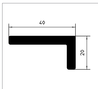
Противоударный защитный профиль Номер материала: 1618254 Материал: RAU-ПВХ 8389
