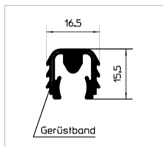
Крепёжная планка
