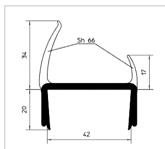
Профиль для уплотнения двери Номер материала: 1630062 (Z) Материал: RAU-ПВХ 1309/6658
