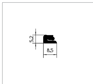
Накладка для подножек Номер материала: 1607610 Материал: RAU-ПВХ 7758
