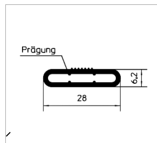
Профиль для поручней
