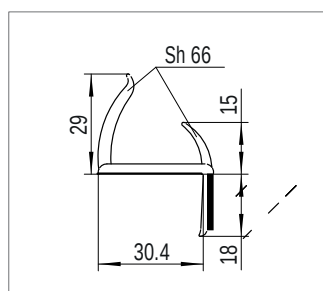
Профиль для уплотнения двери Номер материала: 1625159 Материал: RAU-ПВХ 1103/6656
