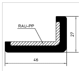
Противоударный защитный профиль Номер материала: 1632833 Материал: RAU-ПП 1381 / TPEV
