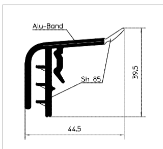
Парапетный профиль
