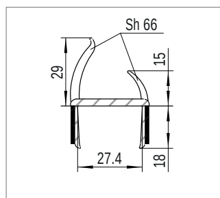
Профиль для уплотнения двери Номер материала: 1638972 (Z) Материал: RAU-ПВХ 1309/6658
