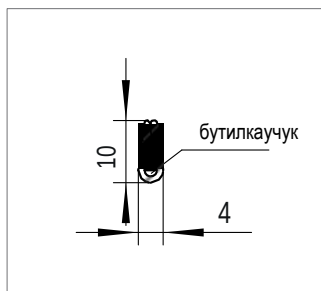
Пароизоляционный профиль Номер материала: 1956841 Материал: RAU-ППМЭ 504
