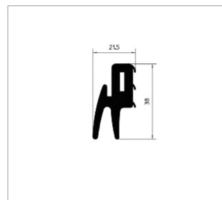
Уплотнительный профиль
