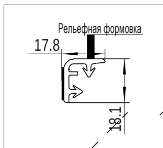
Специальный профиль
