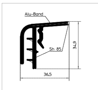
Парапетный профиль
