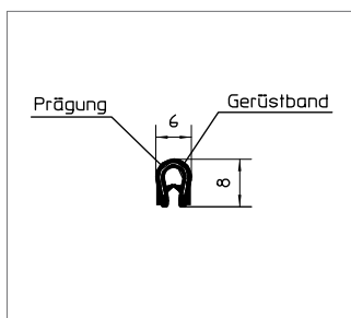
Профиль для защиты кромок армированный металлом Номер материала: 1630172 Материал: RAU-ПВХ 8505
