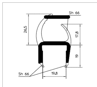
Профиль для уплотнения двери Номер материала: 1609593 Материал: RAU-ПВХ 1309/6658
