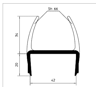
Профиль для уплотнения двери Номер материала: 1632872 Материал: RAU-ПВХ 1309/6658
