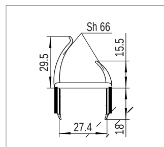
Профиль для уплотнения двери Номер материала: 1616108 Материал: RAU-ПВХ 1103/7558
