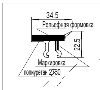
Специальный профиль
