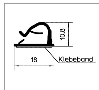
Профиль с клейкой лентой для проводки кабеля
