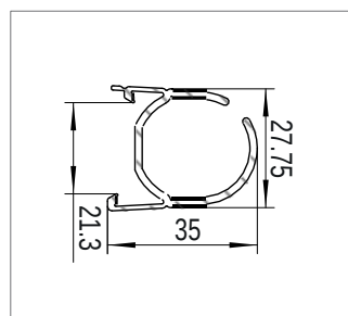
Облицовочный профиль Номер материала: 1617079 Material: RAU-АБС 166
