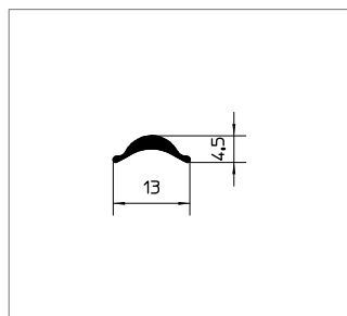
Заполнитель для кромок Номер материала: 1606743 Материал: RAU-ПВХ 8905
