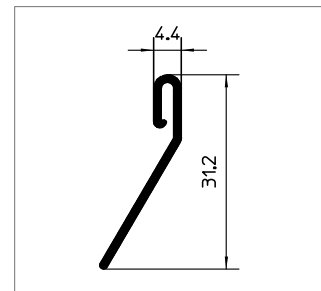
Облицовочный профиль с шарнирной петлёй
