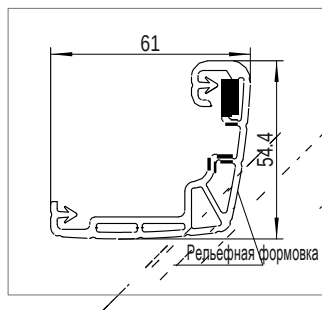
Специальный профиль
