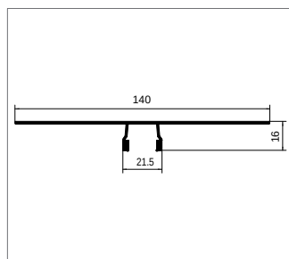
Облицовочный профиль
