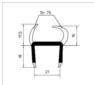
Профиль для уплотнения двери Номер материала: 1610692 Материал: RAU-ПВХ 1309/7558
