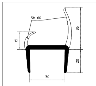
Профиль для уплотнения двери Номер материала: 1605502 Материал: RAU-ПВХ 1309 /6058
