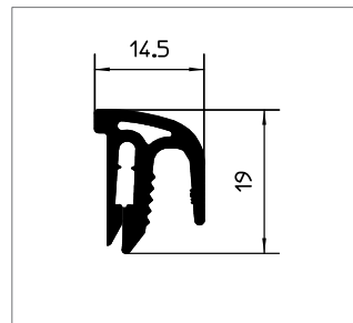
Профиль-герметик для оконной полости двери кузова
