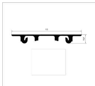
Клеммная планка
