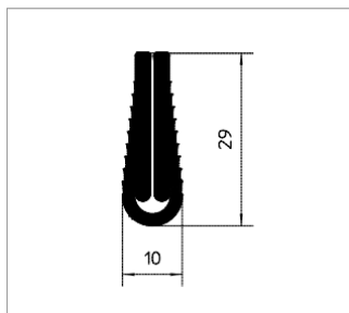
Зажимный профиль Номер материала: 1616283 Материал: RAU-ПВХ 9089
