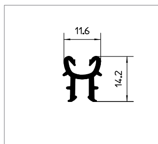
Профиль-вставка
