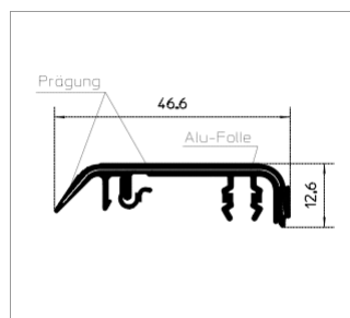
Облицовочный профиль
