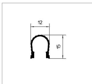
Погружной профиль для вставки Номер материала: 1954646 Материал: RAU-ПА 102
