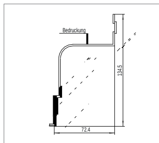
Щиток-грязеотбойник Номер материала: 1625505 Материал: RAU-ПП 234
