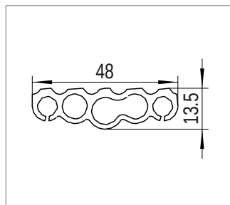
Защитный профиль Номер материала: 1606513 Материал: RAU-ПВХ 8008
