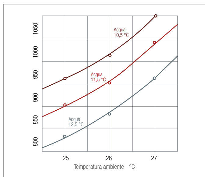
Grafico potenza frigorifera sensibile
