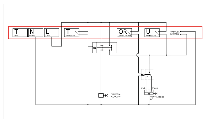
Schema elettrico ecoclima DC
