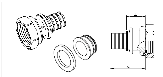
Composizione set raccordo terminale a tenuta piana.
