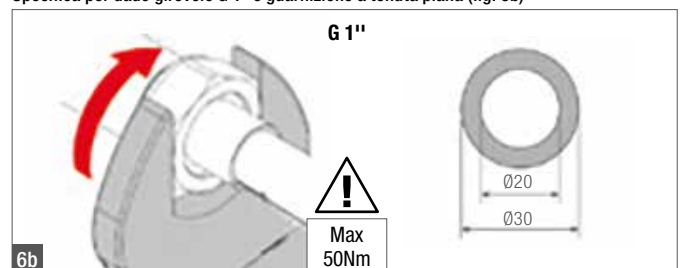
Specifica per dado girevole G 1" e guarnizione a tenuta piana (fig. 6b)
