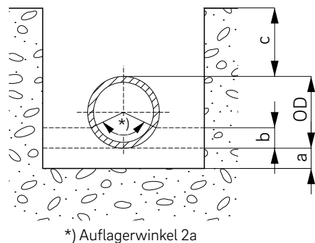
Abb. 05-10 Bettung Typ 1 nach DIN EN 1610
