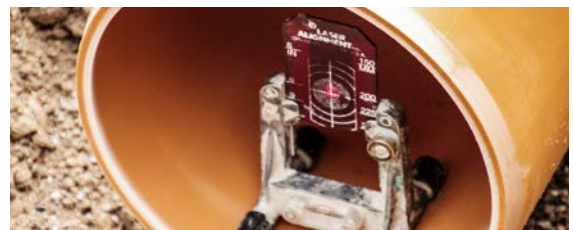
Abb. 05-11 Gefälle-Kontrolle mit einem Laser
