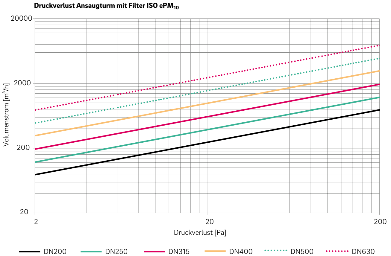
Abb. 08-4 Druckverlust Ansaugturm mit Filter ISO ePM 10
