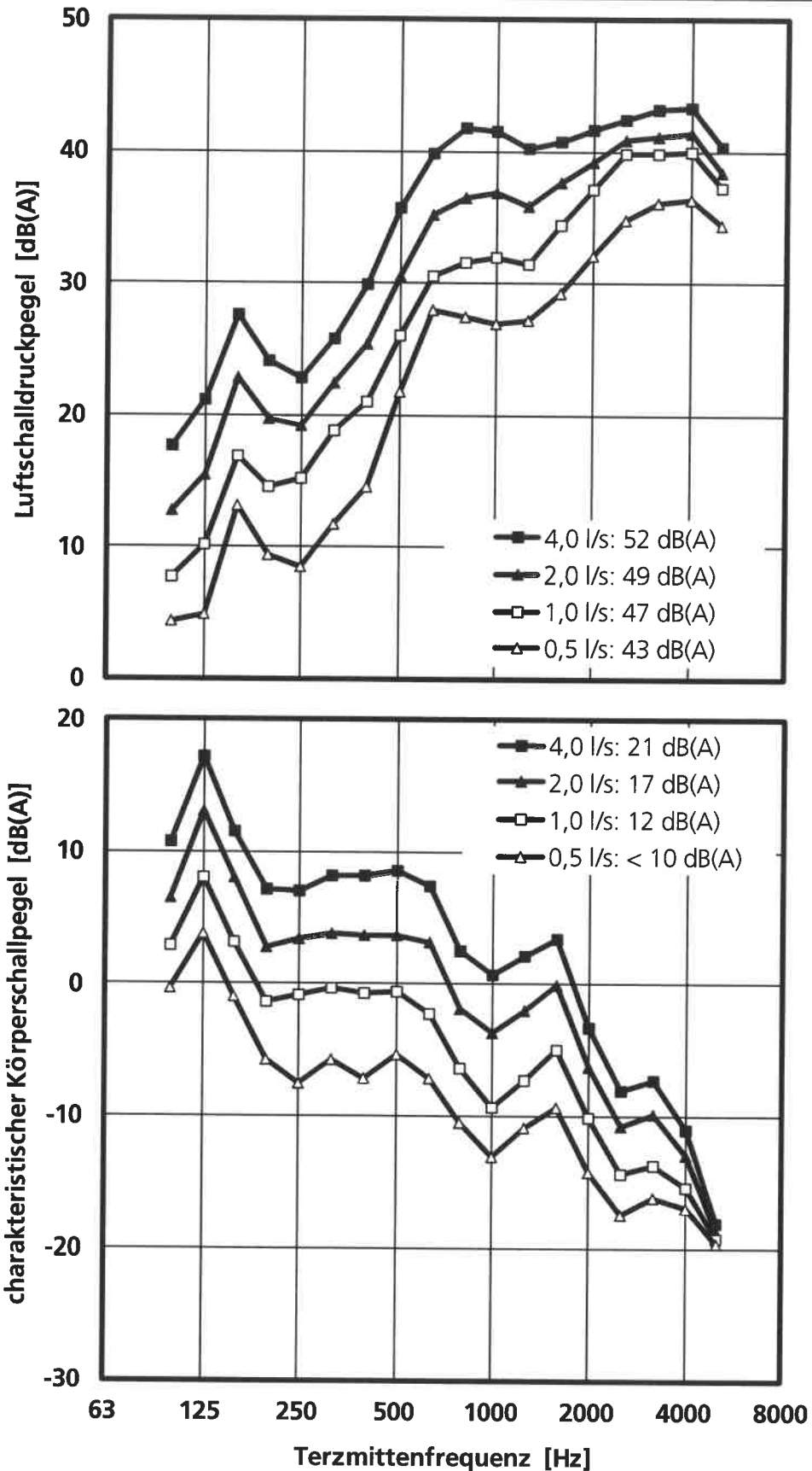
Frequenzspektrum des Luftschalldruckpegels L_{p,A} (oben) und des charakteristischen Körperschallpegels L_{sc,A} (unten) nach DIN EN 14366 bei verschiedenen Volumenströmen.
