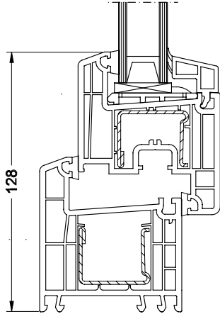
ouvrant droit
