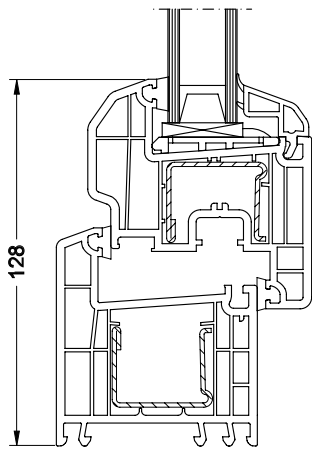
ouvrant « autrichien »
