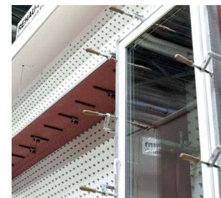
Testovacie zariadenie pre zaťaženie tlakom.
