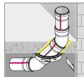
Рис. 74 Косая противопожарная манжета (только для монтажа на потолке)
