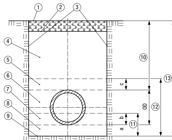
Рис. 89 Схематическое изображение расположения траншей
