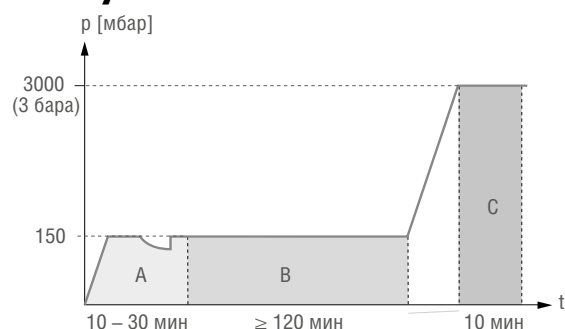
Табл. 19 Диаграмма пневматического испытания A Предварительное испытание (см. табл. 7-1) B Основное испытание C Испытание нагрузкой
