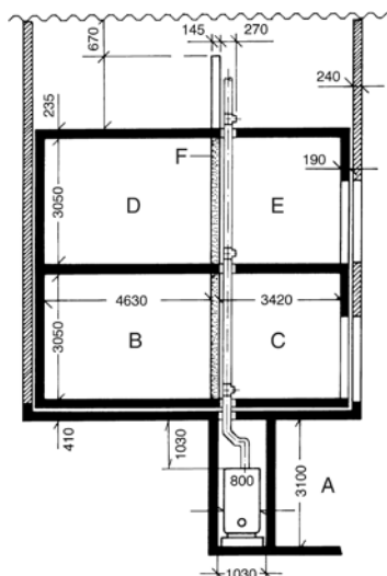
Рис. 68 Испытательный стенд Института строительной физики им. Фраунхофера (все размеры в мм)
