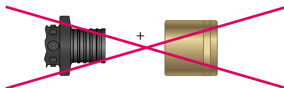
Рис. 16 Недопустимая комбинация фитинга RAUTITAN PX с подвижной гильзой RAUTITAN MX
