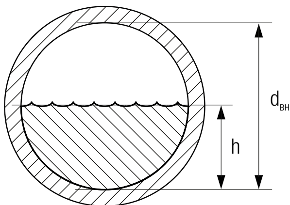
Рис. 91 Поперечный разрез частично наполненного трубопровода d_{BH} Внутренний диаметр трубы h Высота жидкости
