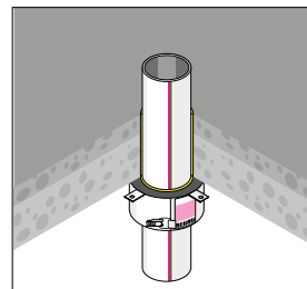
Рис. 72 Монтаж противопожарной манжеты на перекрытии
