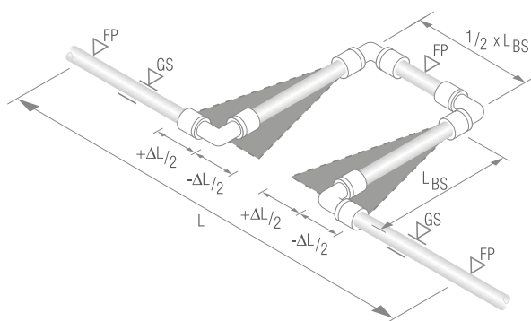
Рис. 32 П-образный компенсатор
