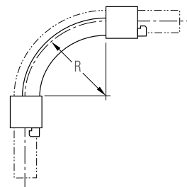
Рис. 44 Фиксаторы поворота (водоснабжение) – 90° и фиксаторы поворота (водоснабжение / отопление) (5 x \varnothing ) – 90° для гнутья труб \varnothing 32
