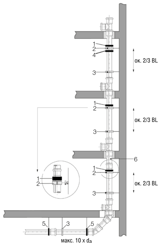
Рис. 87 Схема установки стояка
