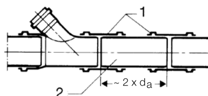
Рис. 77 Установка фасонной части
