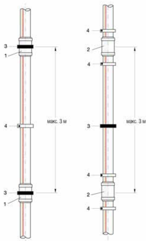
Рис. 76 Применение двухраструбных или надвижных муфт
