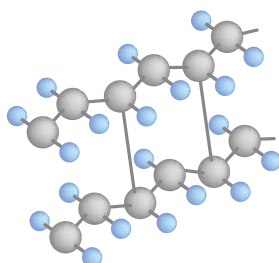
Рис. 8 Сшитый полиэтилен (PE-X)
