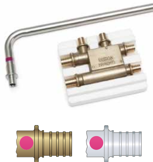
Рис. 20 Отличительные особенности фитингов для систем отопления
