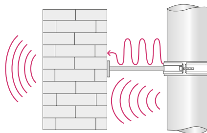
Рис. 66 Распространение шума в канализационных системах
