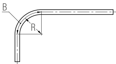
Рис. 46 Обозначение радиуса и длины изгиба R = радиус изгиба B = длина изгиба
