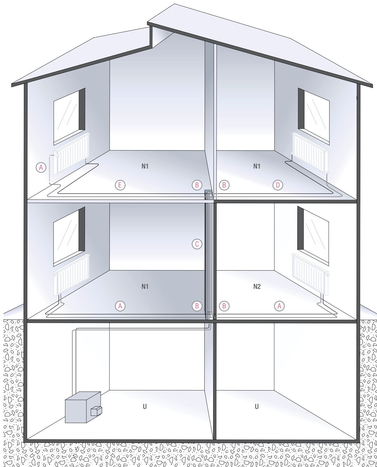
Рис. 27 Монтажные ситуации при изоляции трубопроводов N1 Пользователь 1 N2 Пользователь 2 U Неотапливаемые помещения
