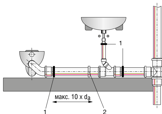
Рис. 88 Схема монтажа горизонтального трубопровода
