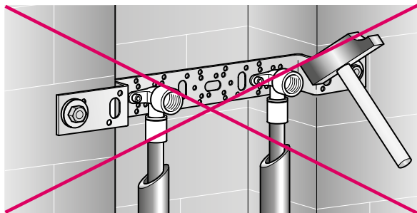
Рис. 53 Не выправлять молотком!
