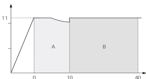
Табл. 17 Диаграмма гидравлического испытания для труб RAUTITAN stabil
