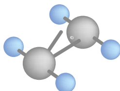
Рис. 6 Этилен, образование свободной связи
