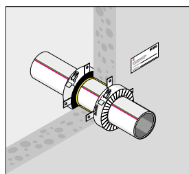
Рис. 73 Монтаж противопожарной манжеты на стене
