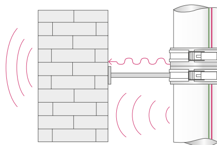
Рис. 67 Снижение шума в системе RAUPIANO PLUS
