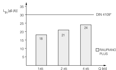
Рис. 70 Результаты измерений системы со стандартным креплением в помещении на нижнем этаже за стеной со стояком (источник: Институт строительной физики им. Фраунхофера, Штутгарт, протокол испытания P-BA 176/2006)
