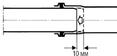
Рис. 75 Выдвинуть трубу из раструба на 10 мм для обеспечения компенсации температурного расширения
