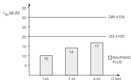
Рис. 69 Результаты измерений системы с крепежными хомутами, снижающими распространение шума через строительные конструкции, в помещении на нижнем этаже за стеной со стояком (источник: Институт строительной физики им. Фраунхофера, Штутгарт, протокол испытания P-BA 6/2006)
