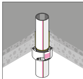
Рис. 71 Монтаж противопожарной манжеты в перекрытие
