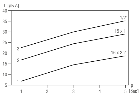
Рис. 30 Результат испытания Института им. Фраунхофера: сравнительный анализ шумоизолирующих характеристик материалов труб
