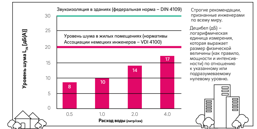
Результаты испытаний для трубы RAUPIANO PLUS
