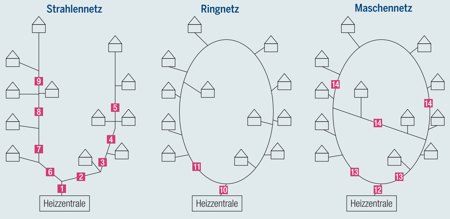
Abb. 1: Die Entscheidung für eine Netzform richtet sich nach den Kosten der Rohre, der Versorgungssicherheit sowie den nachträglichen Erweiterungsmöglichkeiten.
