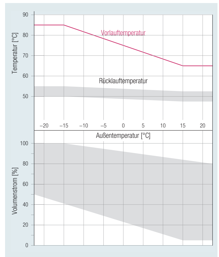
Abb. 2: Netzregelung, kombinierte Fahrweise aus Temperatur- und Mengenregelung
