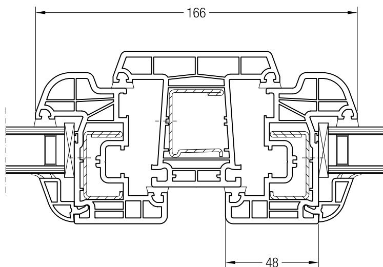
Sloupek 86 BriD s křídlem 48 oblé BriD, 1550481
