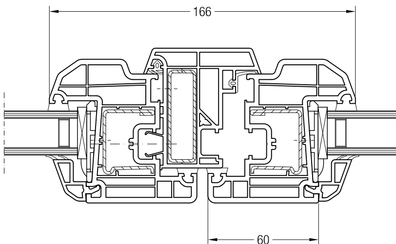
Statická velká klapačka konstrukční hloubky 70 s křídlem A 60 BriD, 1550050
