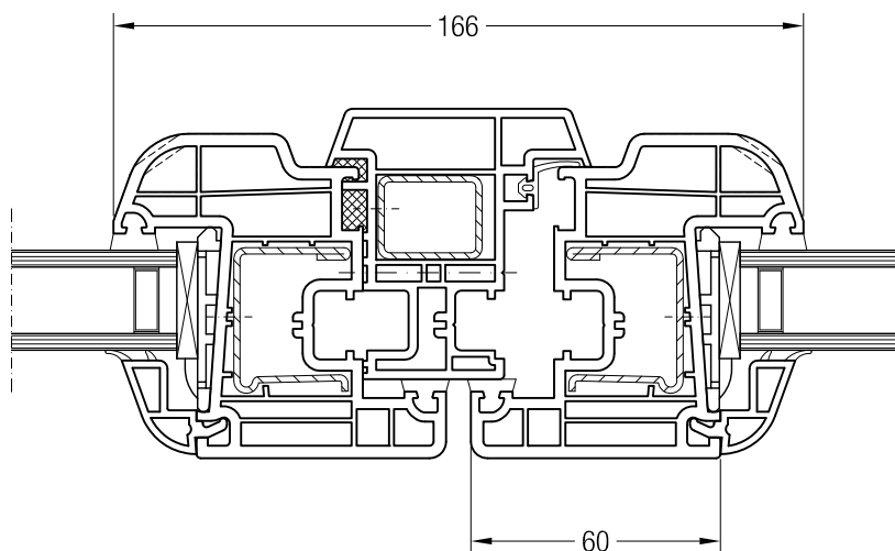
Velká klapačka č. 1/70 s křídlem A 60 BriD, 1550050 nebo s křídlem 60 oblé BriD, 1550060
