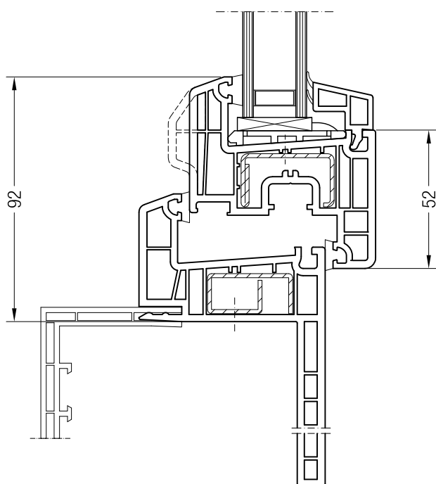
Rám pro rekonstrukce 40 nebo 60 BriD s křídlem Z 52 BriD, 1550480 nebo s křídlem A 52 BriD, 1550040
