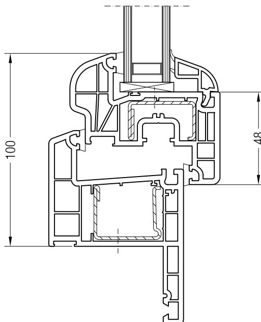
Rám 60/40 BriD s křídlem 48 oblé BriD, 1550481
