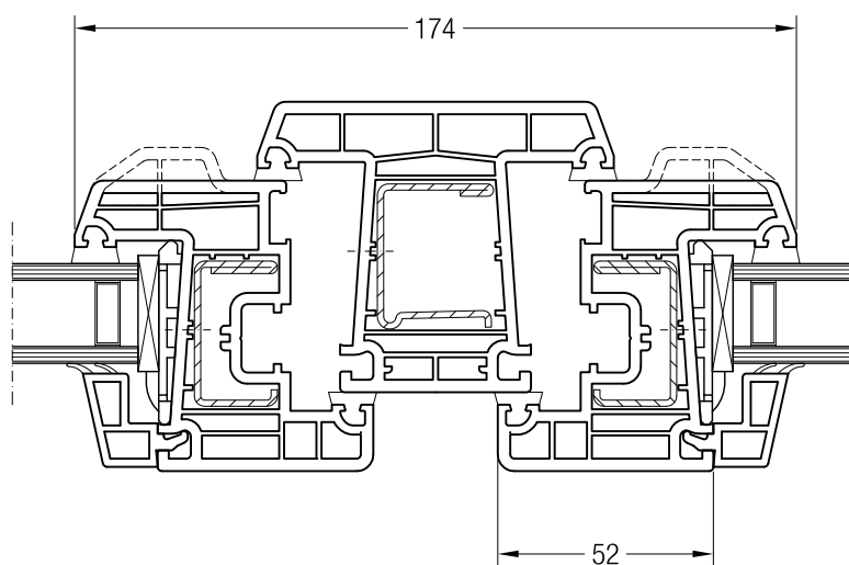
Sloupek 86 BriD s křídlem Z 52 BriD, 1550480 nebo s křídlem A 52 BriD, 1550040
