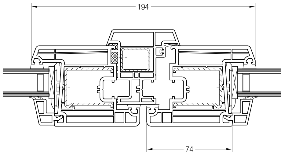
Velká klapačka č. 1/70 s křídlem Z 74 BriD, 1550510
