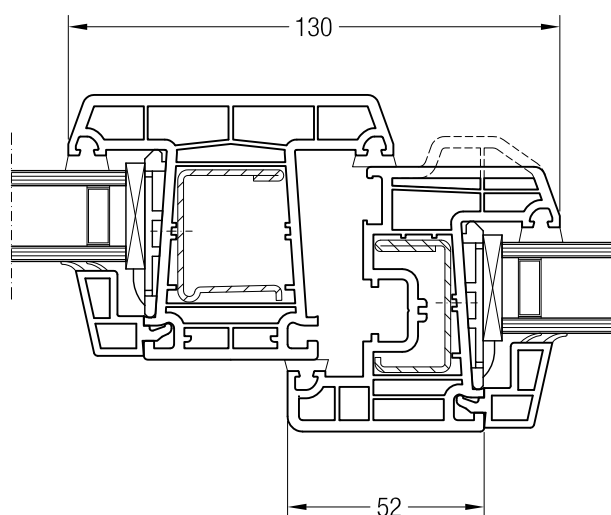
Sloupek 86 BriD s křídlem Z 52 BriD, 1550480 nebo s křídlem A 52 BriD, 1550040
