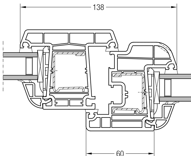
Sloupek 86 BriD s křídlem A 60 BriD, 1550050 nebo s křídlem 60 oblé BriD, 1550060
