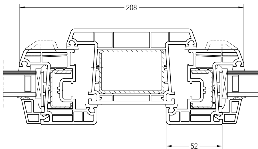
Sloupek 120 BriD s křídlem Z 52 BriD, 1550480 nebo s křídlem A 52 BriD, 1550040
