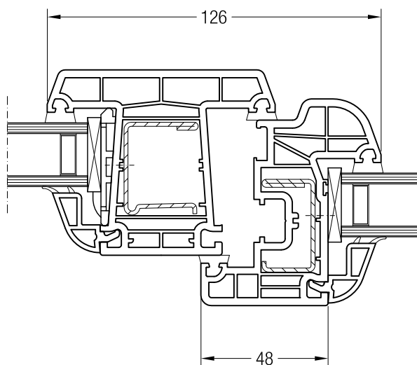
Sloupek 86 BriD s křídlem 48 oblé BriD, 1550481
