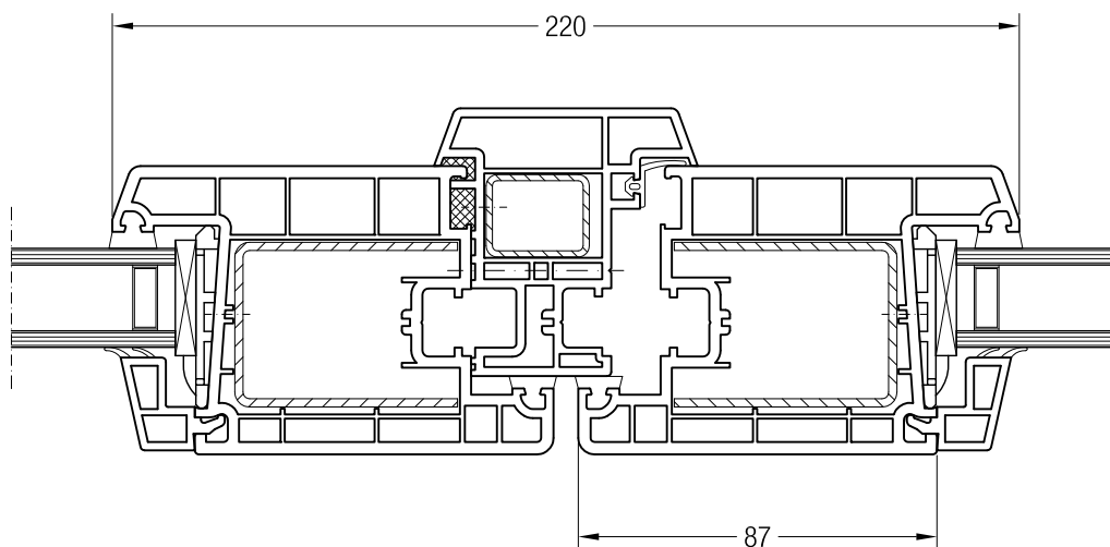
Velká klapačka č. 1/70 s křídlem Z 87 BriD, 1550760
