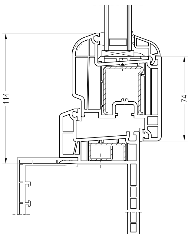
Rám pro rekonstrukce 40 nebo 60 BriD s křídlem A 74 BriD, 1550390 nebo s křídlem 74 oblé BriD, 1550070
