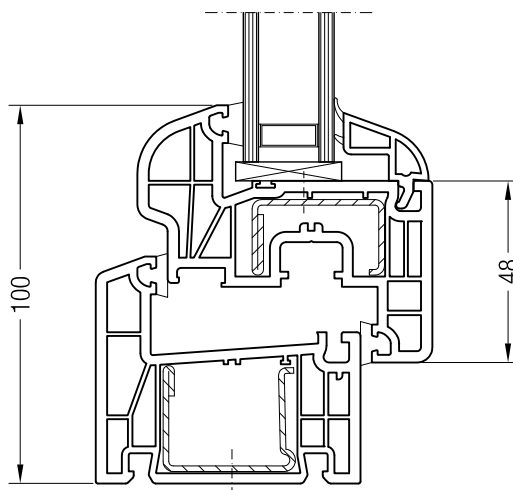
Rám 60 DK BriD s křídlem 48 oblé BriD, 1550481
