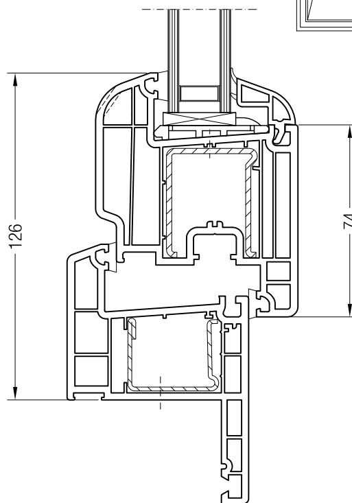
Rám 60/40 BriD s křídlem A 74 BriD, 1550390 nebo s křídlem 74 oblé BriD, 1550070
