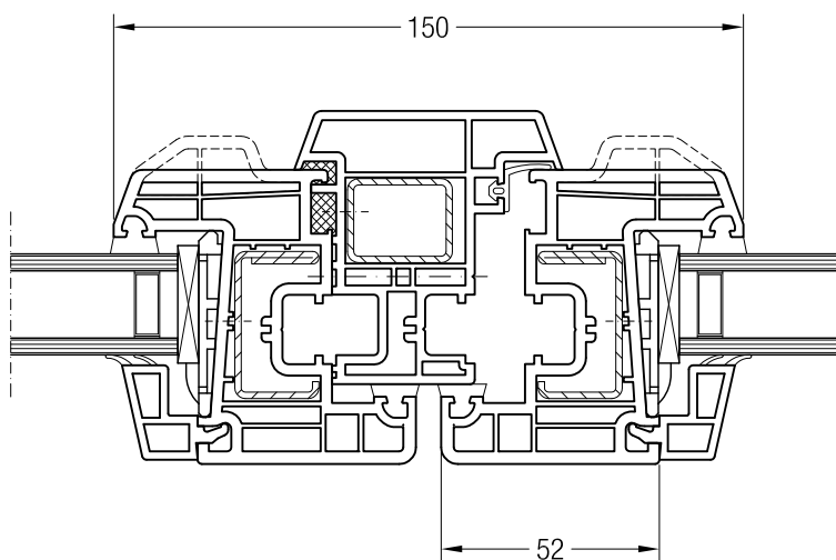
Velká klapačka č. 1/70 s křídlem Z 52 BriD, 1550480 nebo s křídlem A 52 BriD, 1550040
