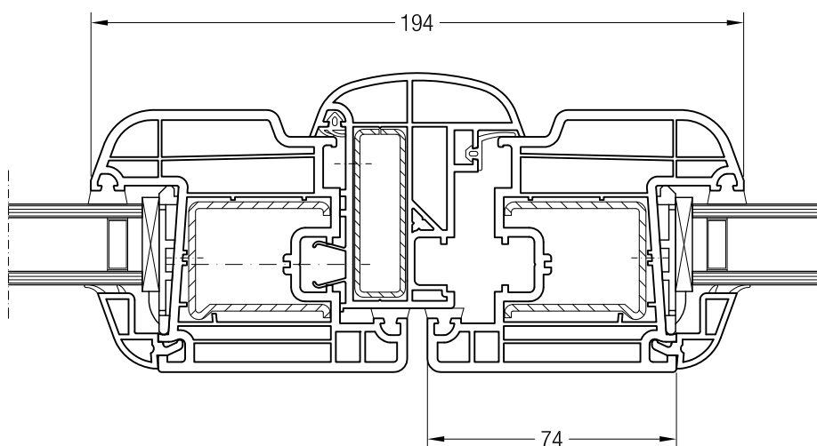
Velká oblá klapačka konstrukční hloubky 70 s křídlem 74 oblé BriD, 1550070
