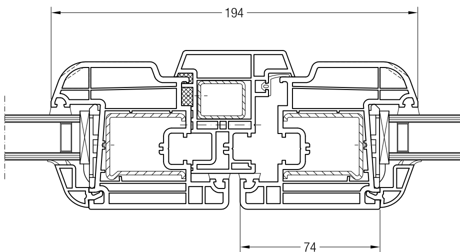
Velká klapačka č. 1/70 s křídlem A 74 BriD, 1550390 nebo s křídlem 74 oblé BriD, 1550070
