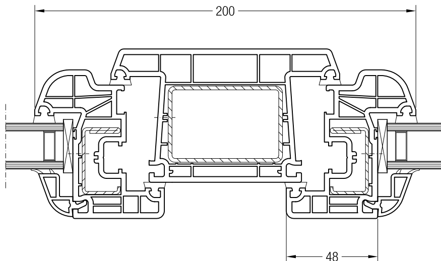
Sloupek 120 BriD s křídlem 48 oblé BriD, 1550481
