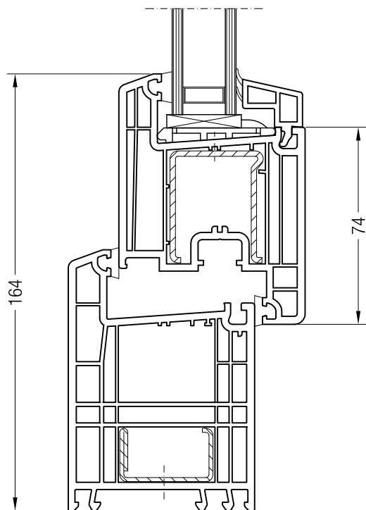
Rám 98 BriD s křídlem Z 74 BriD, 1550510
