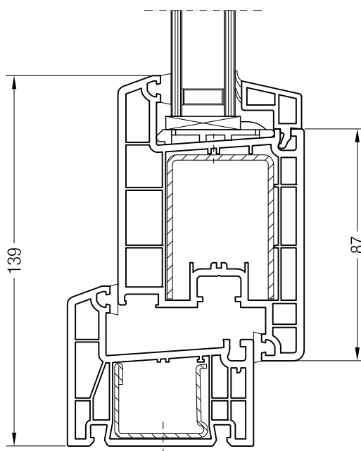
Rám 60 DK BriD s křídlem Z 87 BriD, 1550760
