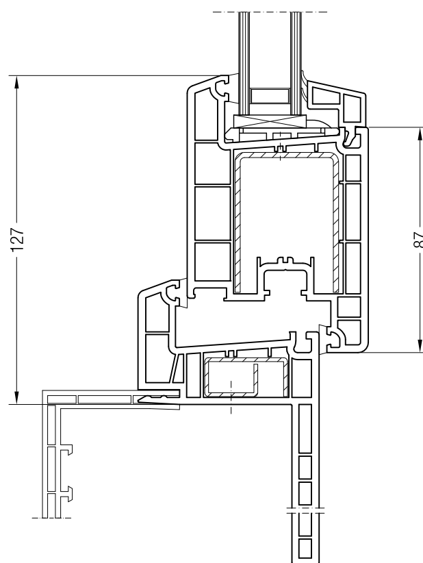
Rám pro rekonstrukce 40 nebo 60 BriD s křídlem Z 87 BriD, 1550760
