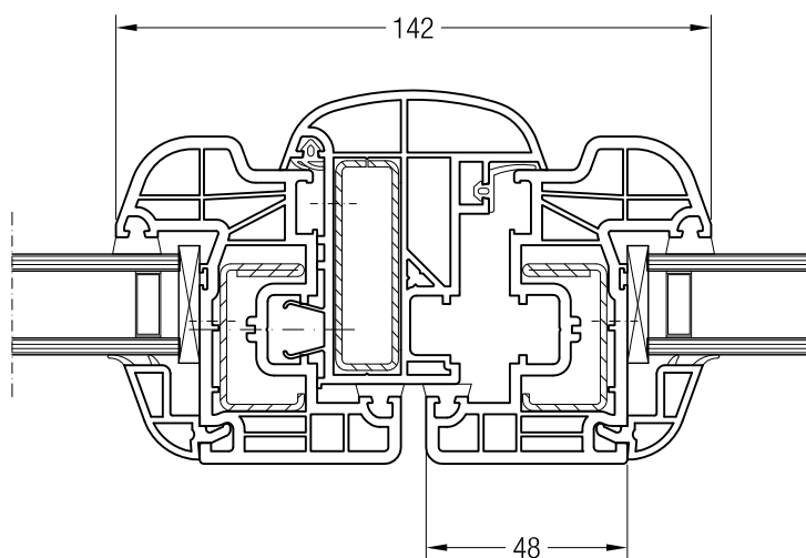
Velká oblá klapačka konstrukční hloubky 70 s křídlem 48 oblé BriD, 1550481
