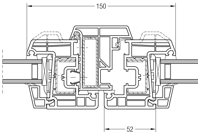
Statická velká klapačka konstrukční hloubky 70 s křídlem Z 52 BriD, 1550480 nebo s křídlem A 52 BriD, 1550040
