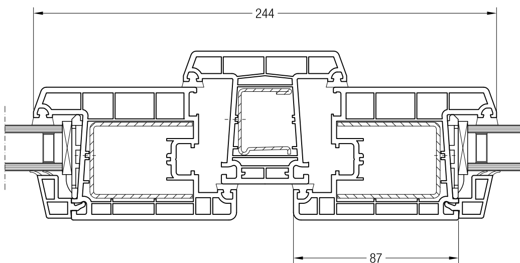
Sloupek 86 BriD s křídlem Z 87 BriD, 1550760
