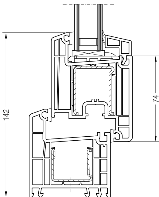
Rám 76-2 BriD s křídlem Z 74 BriD, 1550510
