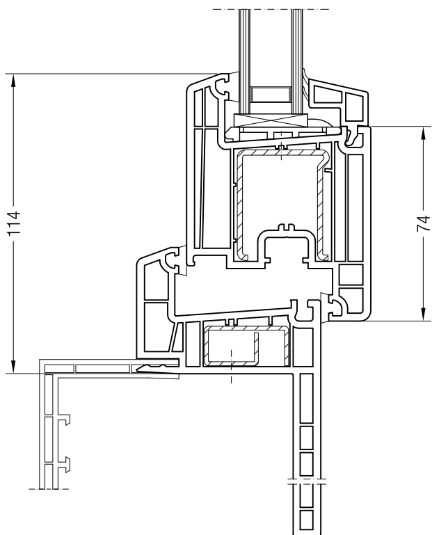
Rám pro rekonstrukce 40 nebo 60 BriD s křídlem Z 74 BriD, 1550510
