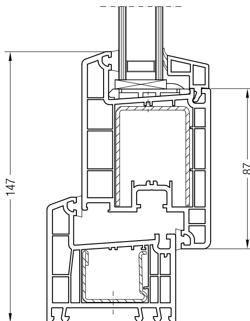
Rám 68 BriD s křídlem Z 87 BriD, 1550760
