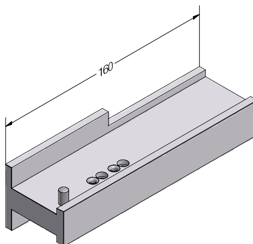
Vrtací šablona sloupku/poutce konstrukční hloubky 70
