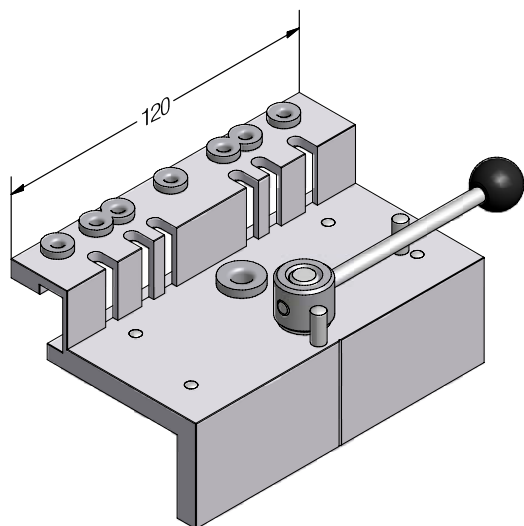
Vrtací šablona rámu konstrukční hloubky 70
