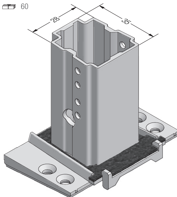
Mechanický spojovač ZDG sloupku 86 konstrukční hloubky 70
