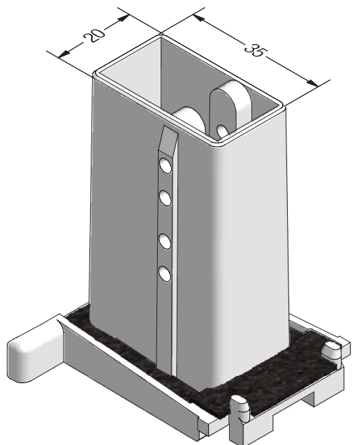
Mechanický spojovač sloupku 78 ED70
