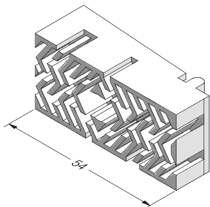
Těsnící díl pro univerzální dveřní práh konstrukční hloubky 70
