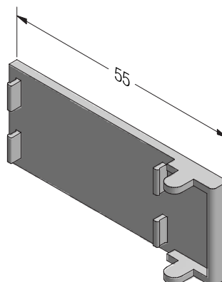
Krytka držáku prahu univerzálního dveřního prahu konstrukční hloubky 70
