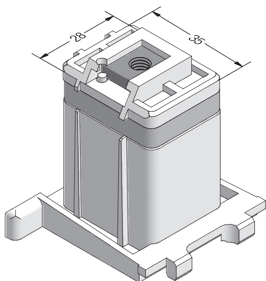
Mechanický spojovač č. 2 sloupku 86 konstrukční hloubky 70
