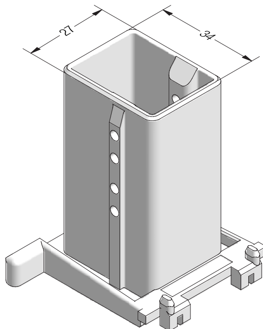
Mechanický spojovač č. 1 sloupku 86 konstrukční hloubky 70
