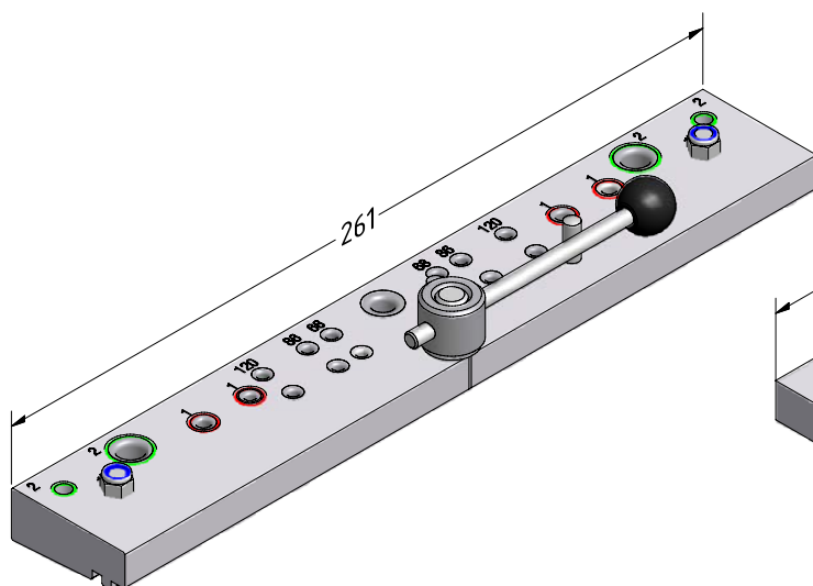
Vrtací šablona kovových spojovačů konstrukční hloubky 70
