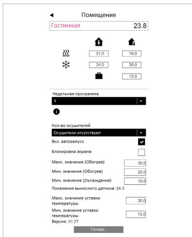
Abb. 8-6 Веб-страница: «Расширенные настройки помещения»
