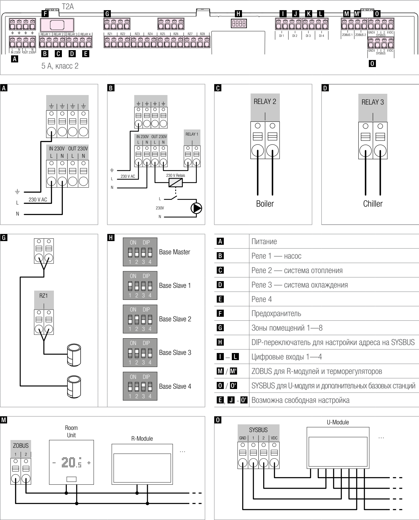
Abb. 10-2 Назначение клемм — базовая станция NEA SMART 2.0 230 В
