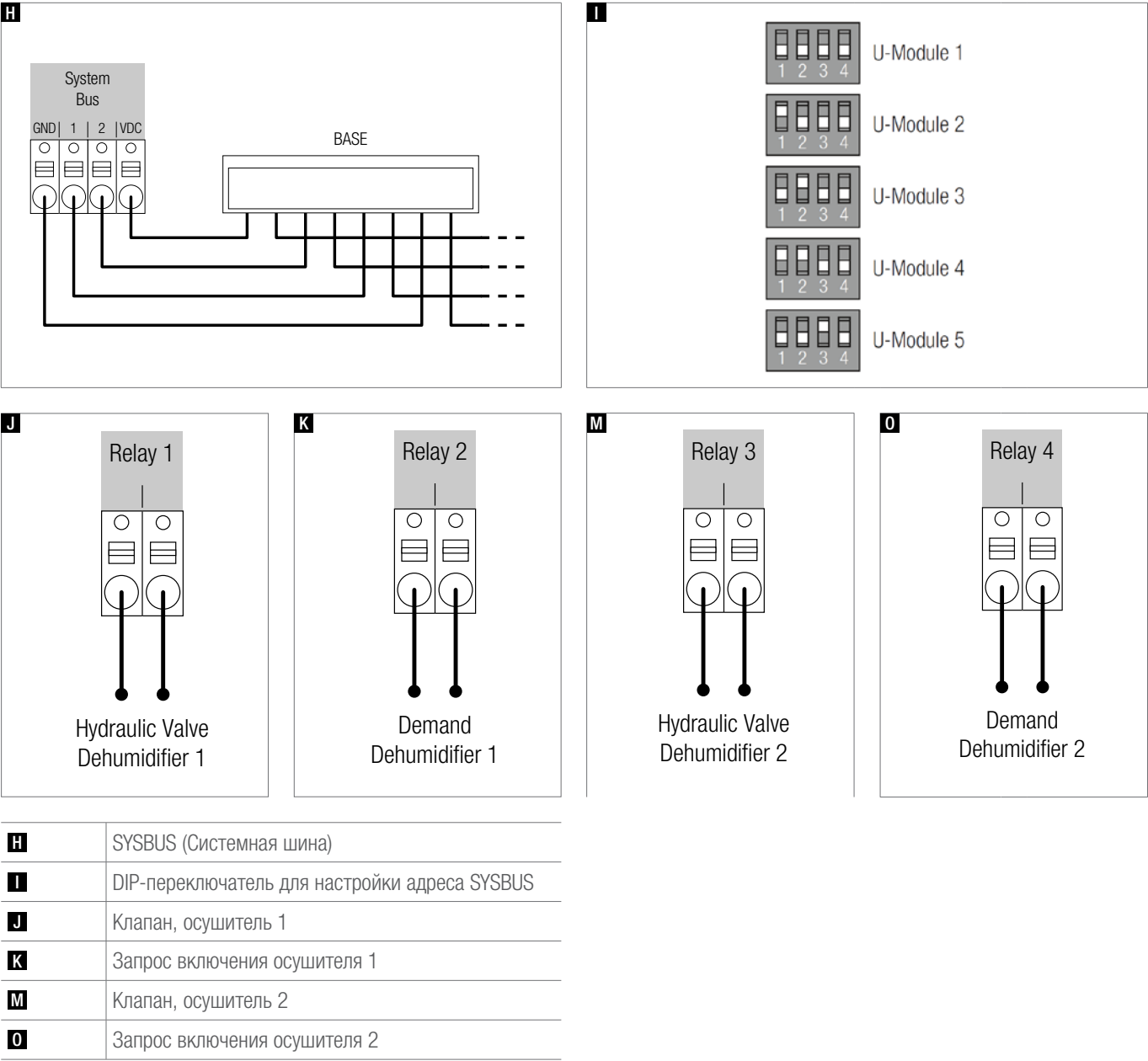
Abb. 10-7 Назначение клемм — U-модуль NEA SMART 2.0 24 В —осушитель
