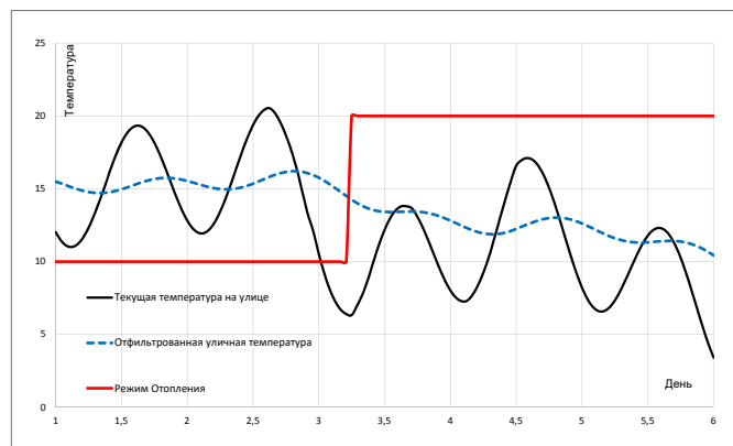
Abb. 4-1 Запуск режима отопления по фильтрованной наружной температуре
