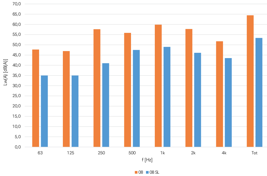
LW(A) Monoblocco Easy Pump 08 Monoblocco Easy Pump 08 SL08 [dB(A)]
