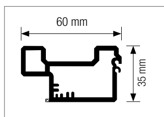
Griffleiste PP mit Eingriff 60 mm
