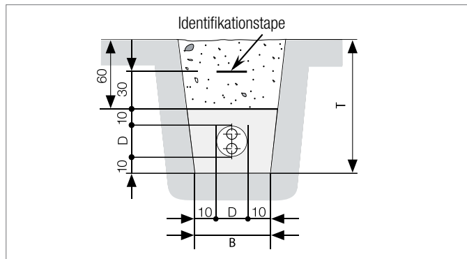
Fig. 34 DUO rørrender
