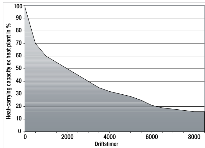
Fig. 20 Årlig tidsskurve
