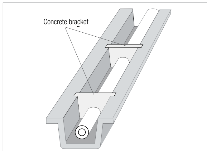
Fig. 39 Jordarbejde
