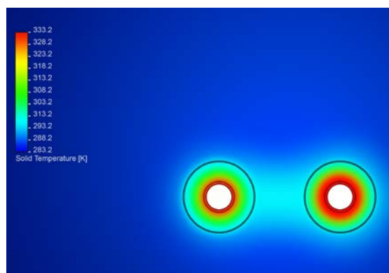
Fig. 27 Varmefordeling ved UNO rør
