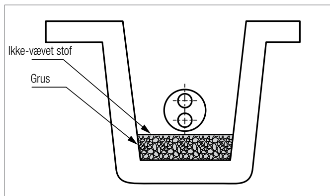
Fig.38 Jordarbejde
