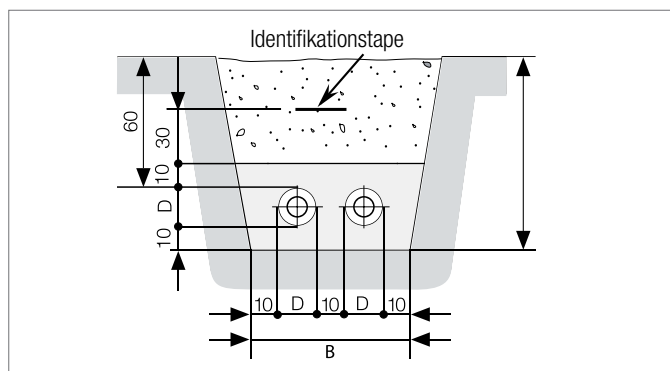
Fig. 35 Rørsystem med UNO rør
