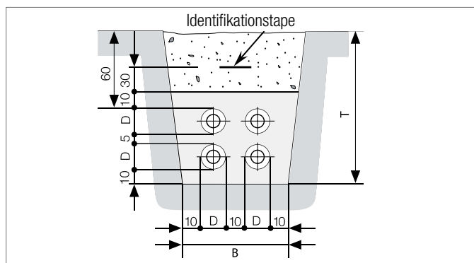
Fig. 36 Rørsystem med UNO rør lagt oven på hinanden
