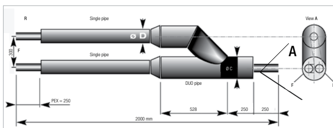
Fig. 55b Overgang fra UNO til DUO rør ved anvendelse af præfabrikeret Y-rør
