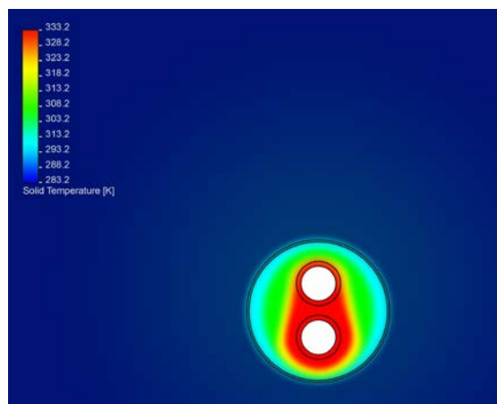
Fig. 28 Varmefordeling ved DUO rør
