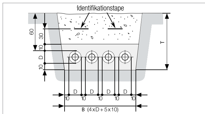
Fig. 37 Rørsystem med UNO rør lagt ved siden af hinanden
