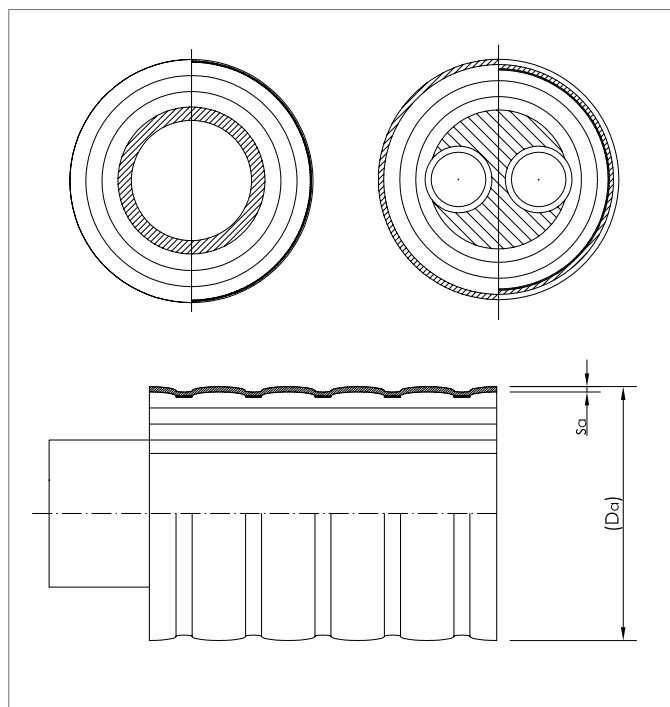
Fig. 16 RAUVITHERM oversigtsdiagram
