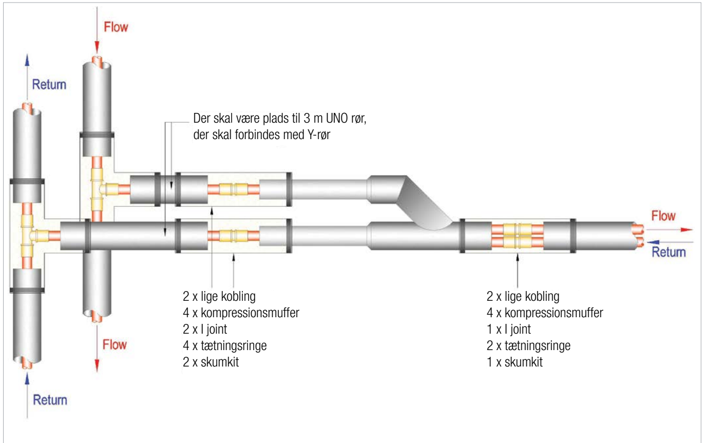
Fig. 55a Overgang fra UNO til DUO rør ved anvendelse af præfabrikeret Y-rør
