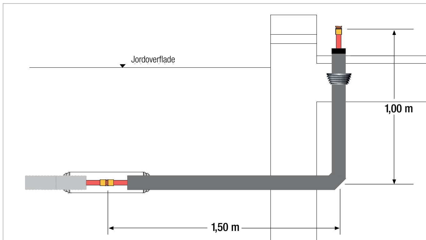
Fig. 54 Installation af præfabrikeret bøjning
