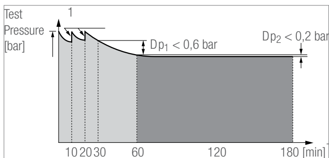
Fig. 60 Tryktest-diagram iht. DIN 1988
