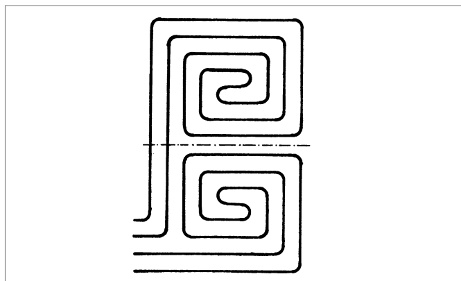
Sl. 4-3 Pravilan raspored fuga kod grejnih krugova
