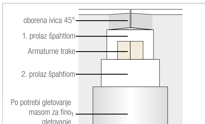
Sl. 5-37 Gletovanje sa armaturnim trakama
