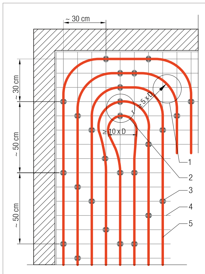
Sl. 4-134 Zaokretne petlje i preusmeravanje u grejnom registru, primer polaganja RAUTHERM S 17 x 2,0 VA 100 mm na RTM 100
