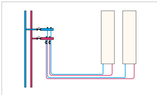
Sl. 5-42 Šematski prikaz odvojenog povezivanja
