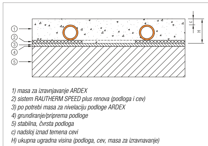
Sl. 4-90 Crtež poprečnog preseka za RAUTHERM SPEED plus renova
