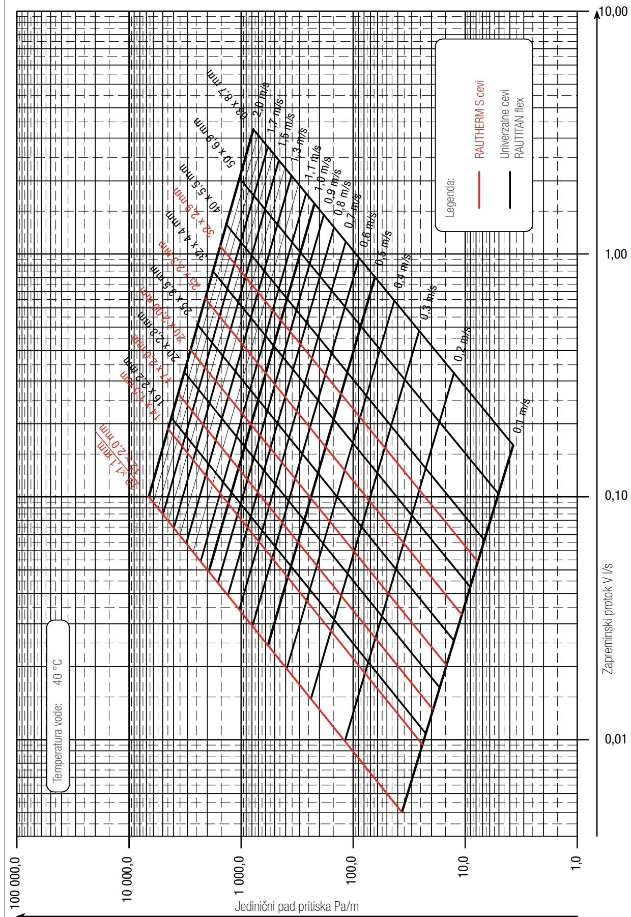
Sl. 5-31 Dijagram pada pritiska za RAUTHERM S i RAUTITAN flex
