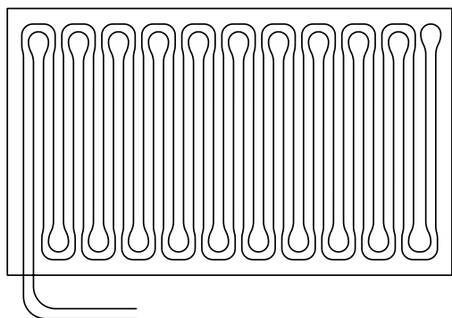
Sl. 5-1 Rashladni plafoni za suhu gradnju
