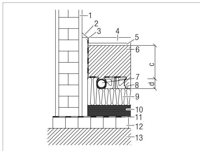
Sl. 4-21 Pečurkasta ploča Varionova sa postavljenom RAUTHERM grejnom cev
