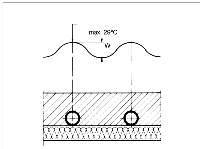
Sl. 16-1 Oscilovanje
