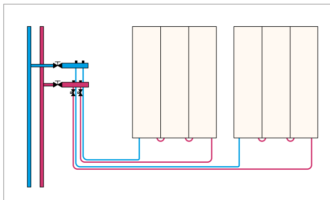
Sl. 5-43 Šematski prikaz serijskog povezivanja
