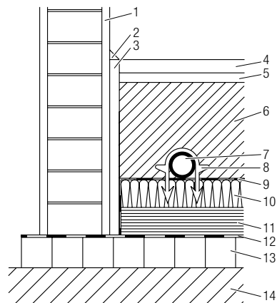
Sl. 4-36 Tacker-ploča BASIC sa Tacker-iglom za pričvršćivanje grejnih cevi
