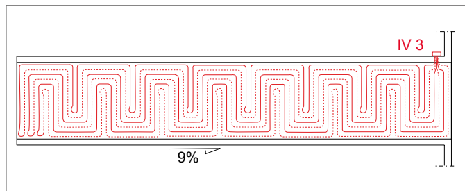
Sl. 12-2 REHAU grejanje površina na otvorenom – grejanje rampe (skica polaganja)
