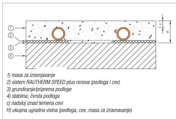
Sl. 4-93 Crtež poprečnog preseka za RAUTHERM SPEED plus renova
