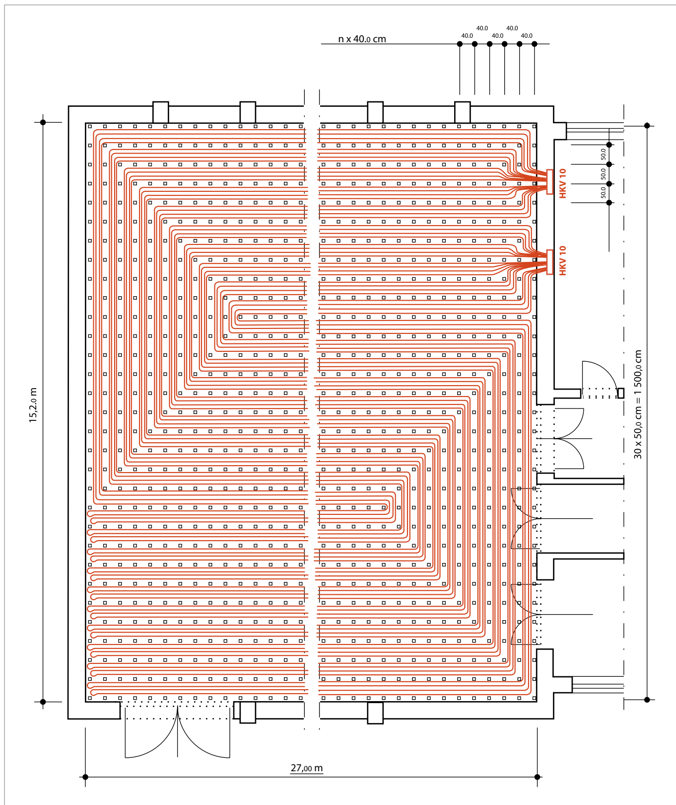
SI. 11-18 REHAU grejanje plivajućih podova, sistem standardni razdelnik
