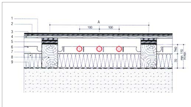
Sl. 11-24 Konstrukcija grejanja plivajućih podova
