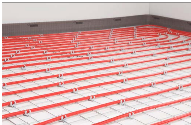
Sl. 4-121 Sistem rešetkaste podloge za polaganje cevi
