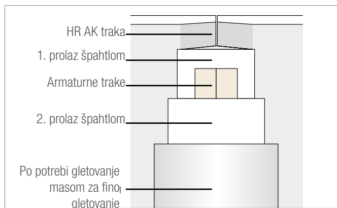
Sl. 5-7 Gletovanje sa armaturnim trakama
