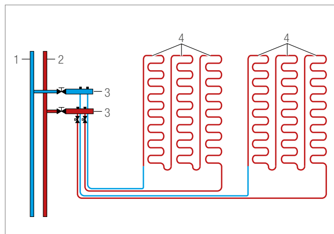
Sl. 5-29 Šematski prikaz serijskog povezivanja više polja zidnog grejanja
