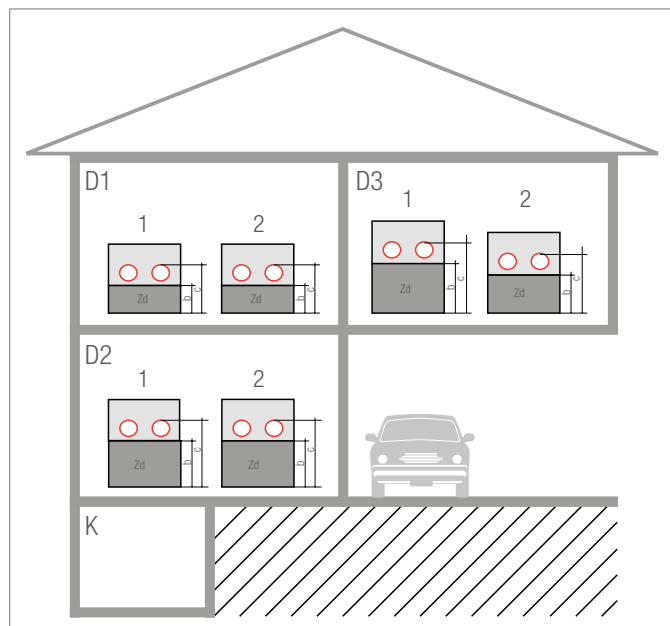
Sl. 4-119 Minimalne konstrukcije izolacionih slojeva kod sistema RAUFIX
