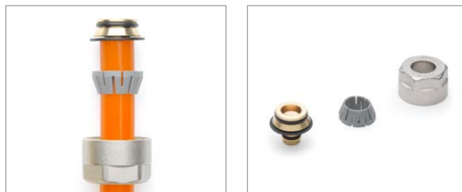
Sl. 4-107 Holender sa steznim prstenom za REHAU cev RAUTHERM SPEED 10 x 1,1 K i 14 x 1,5 K
