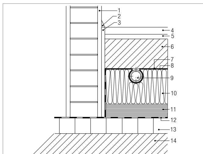
Sl. 4-157 Sistem osnovne ploče TS- 14 sa umetnutom REHAU grejnom cevi
