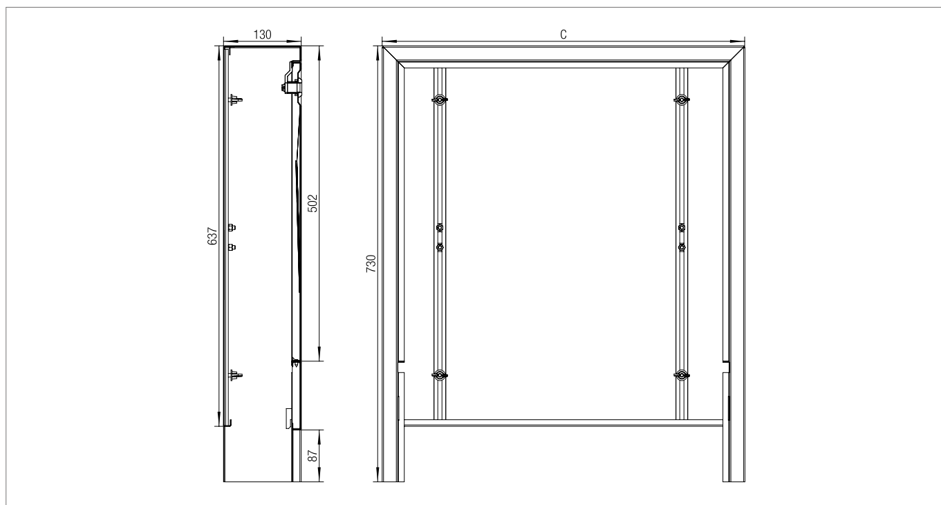
Sl. 7-12 Dimenzije razvodnog ormara AP 130 C Ukupna širina ormara
