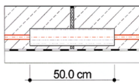
Sl. 10-11 Netiplovana dilataciona fuga sa zaštitom posredstvom 100%-izolacionog creva
