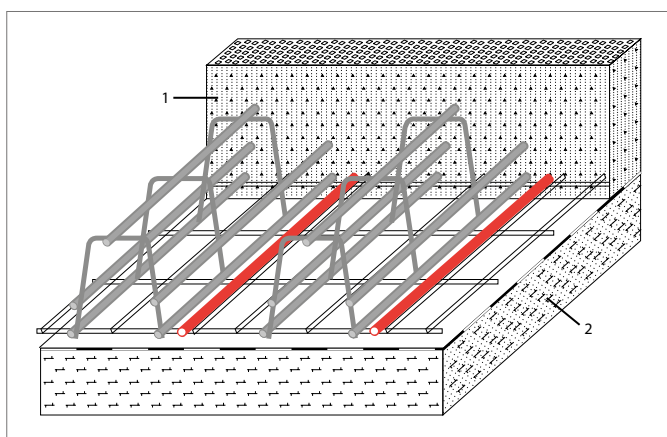
Sl. 10-9 Čeličnim podlogama armirana podna ploča; standardna konstrukcija grejne cevi montirane na donjem sloju armature
