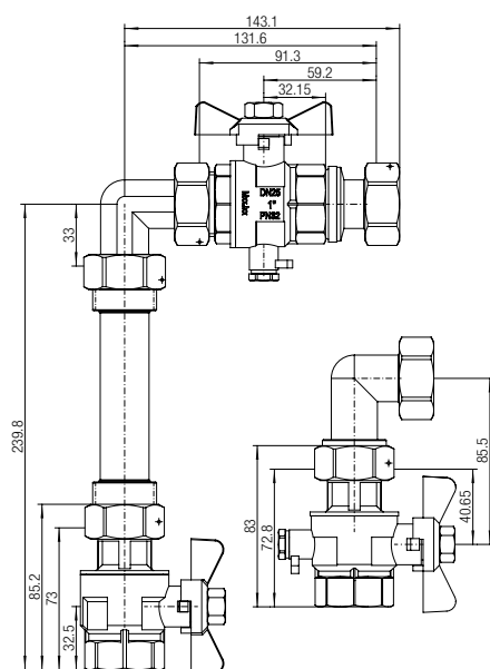
Sl. 7-17 Dimenzije ugradnog seta WMZ, vertikalno
