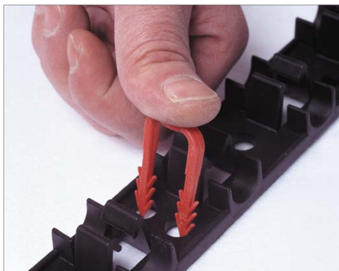
Sl. 4-118 Pritisnuti REHAU pričvrсну iglu u podnu oblogu
