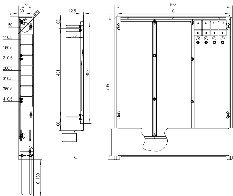
Sl. 7-14 Dimenzije razvodnog ormara UP 75 mm C Širina kućišta iznutra
