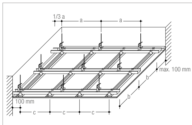
Sl. 5-4 Viseća metalna potkonstrukcija prema DIN 18181 Priključci na zid, vidi Sl. 1-9
