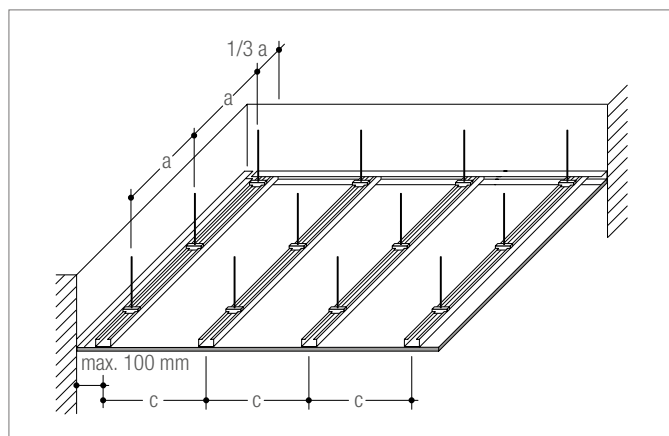
Sl. 5-3 Direktno učvršćena metalna potkonstrukcija prema DIN 18181 Priključci na zid, vidi Abb. 1-9
