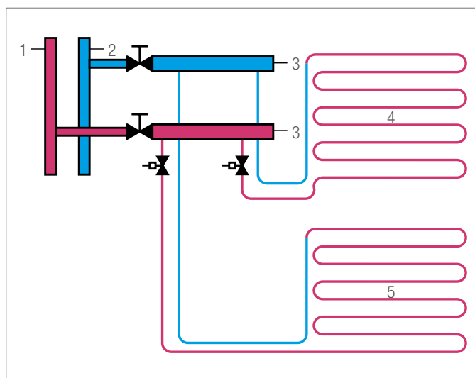
Sl. 5-28 Šematski prikaz odvojenog povezivanja svakog zasebnog polja plafonskog, odn. zidnog grejanja
