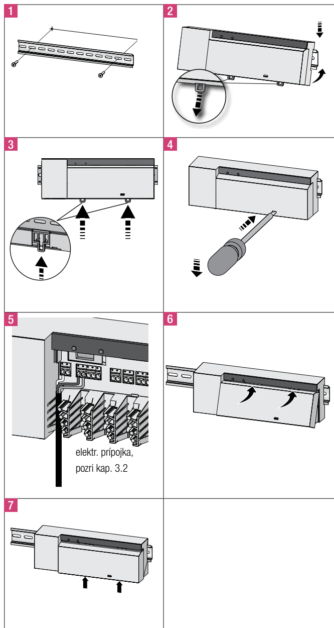
Obr. 3-1 Inštalácia
