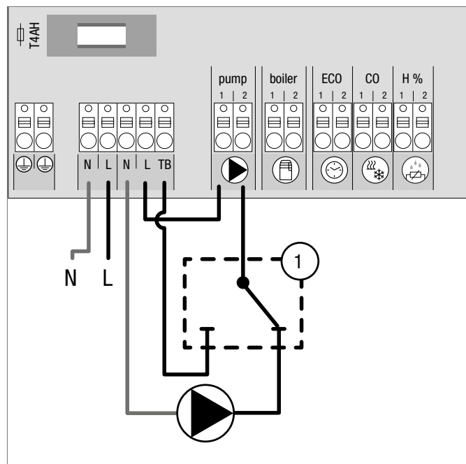
Fig. 3-9 Racordarea unui termostat de limitare
