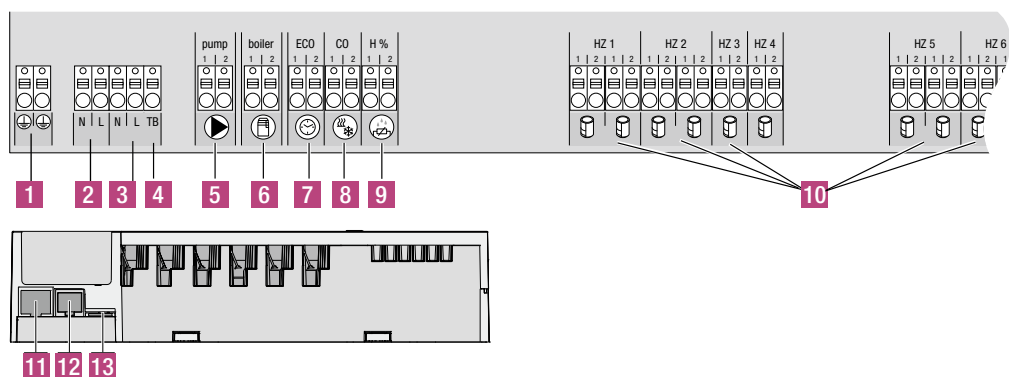
Fig. 2-3 Conexiuni electrice
