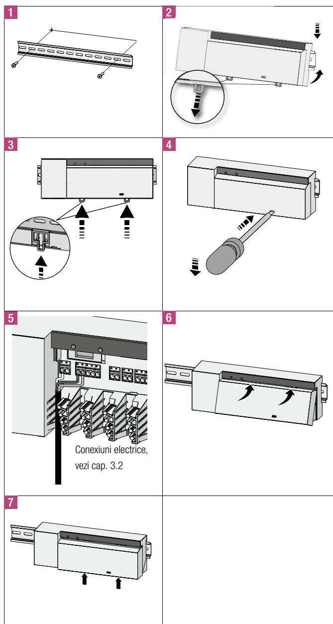
Fig. 3-1 Instalare
