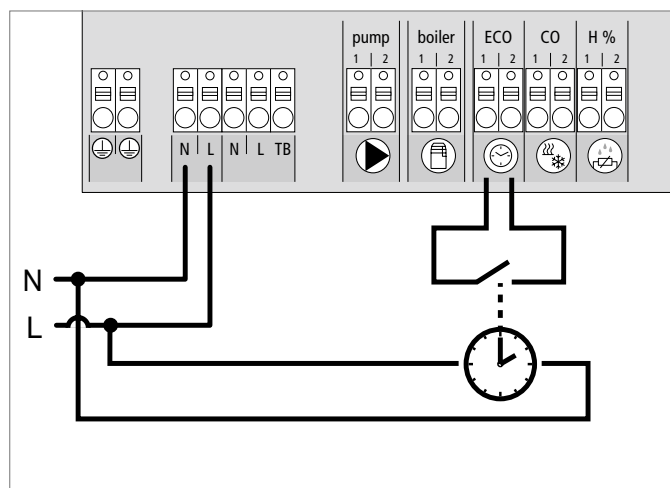
Fig. 3-7 Racordarea unui comutator temporizat extern
