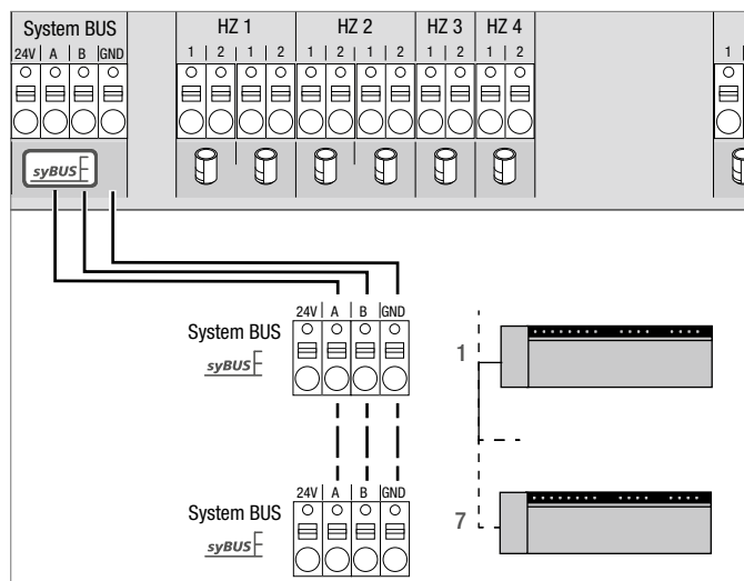
Fig. 3-8 Conectarea stațiilor de bază prin System BUS
