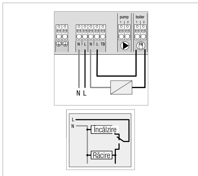
Fig. 3-6 Utilizarea ieșirii „Cazan” ca semnal Pilot pentru Change Over
