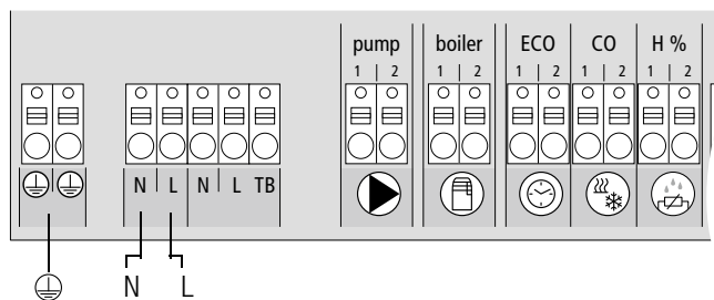
Fig. 3-2 Conexiuni electrice
