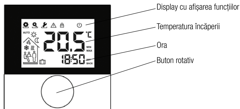
Fig. 4-1 Vedere frontală termostat de cameră Nea Smart D
