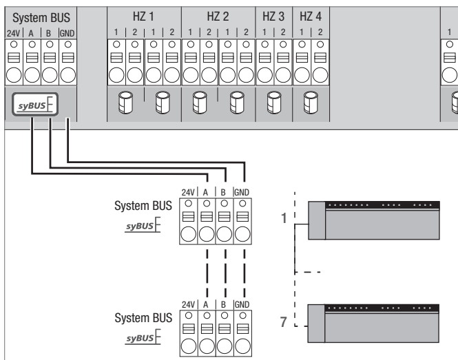
Fig. 3-8 Conexión de la estación base a través del sistema BUS
