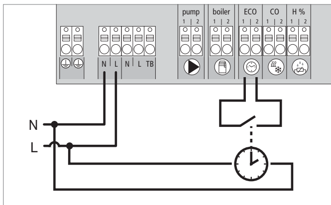
Fig. 3-7 Conexión de un temporizador externo
