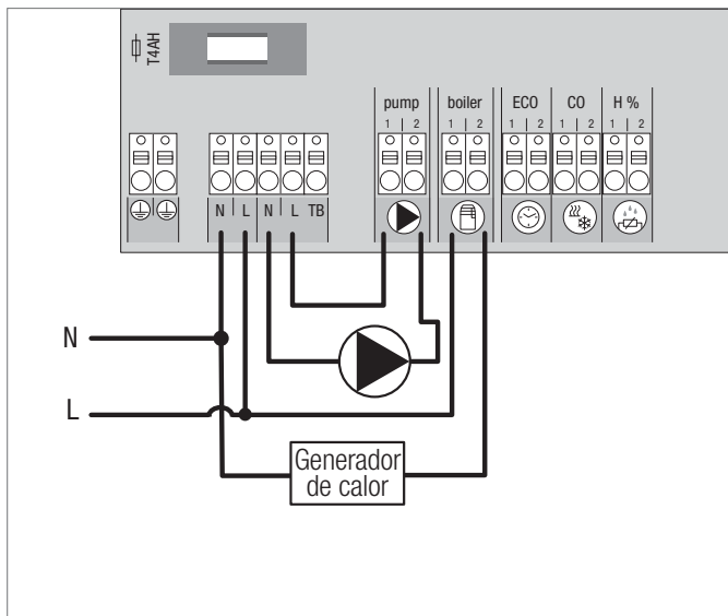
Fig. 3-4 Conexión bomba y caldera
