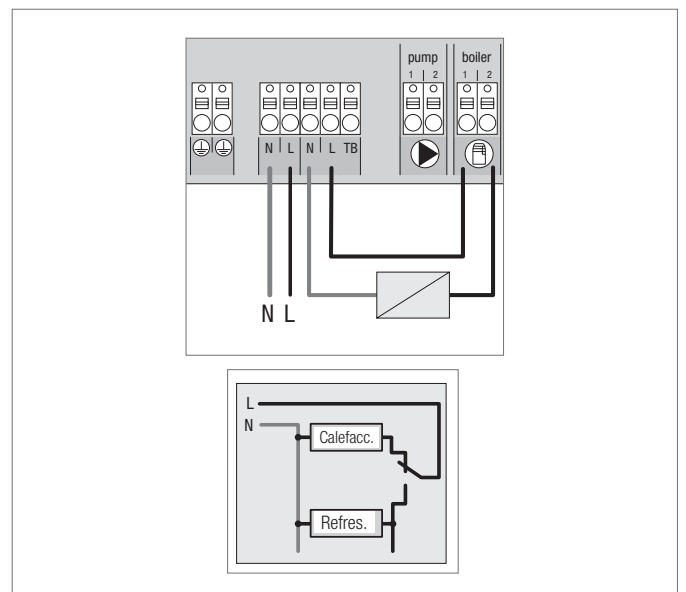
Fig. 3-6 Conmutar el sistema de función de piloto para el Cahnge Over
