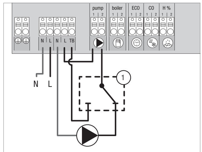
Fig. 3-9 Conexión de un limitador de seguridad de temperatura
