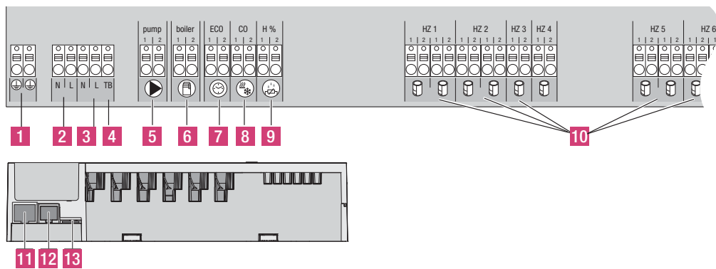
Fig. 2-3 Conexiones
