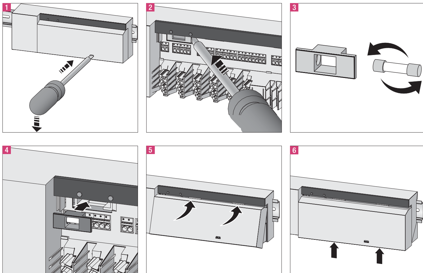
Fig. 6-3 Reemplazo de fusibles
