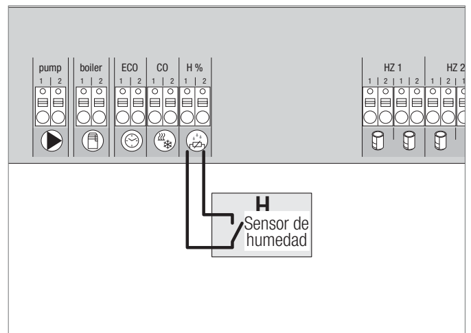
Fig. 3-5 Conexión sensor de humedad
