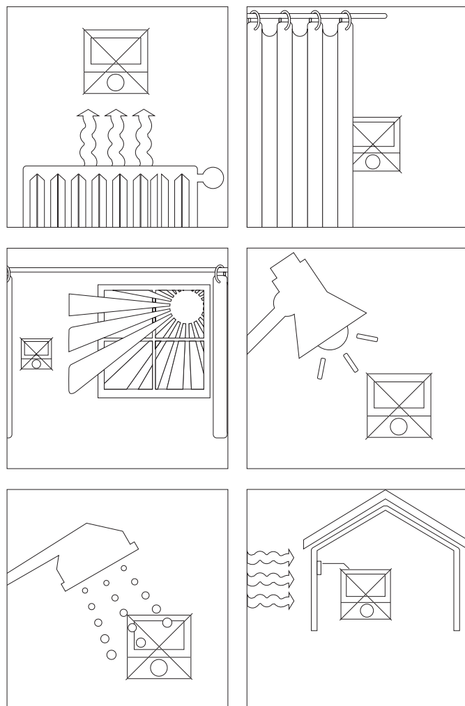
Fig. 3-2 Posiciones de instalación del termostato ambiente
