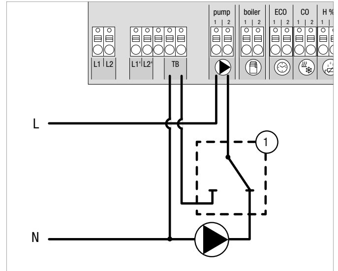
Şek. 3-10 Bir kısıtlama termostatının bağlantısı
