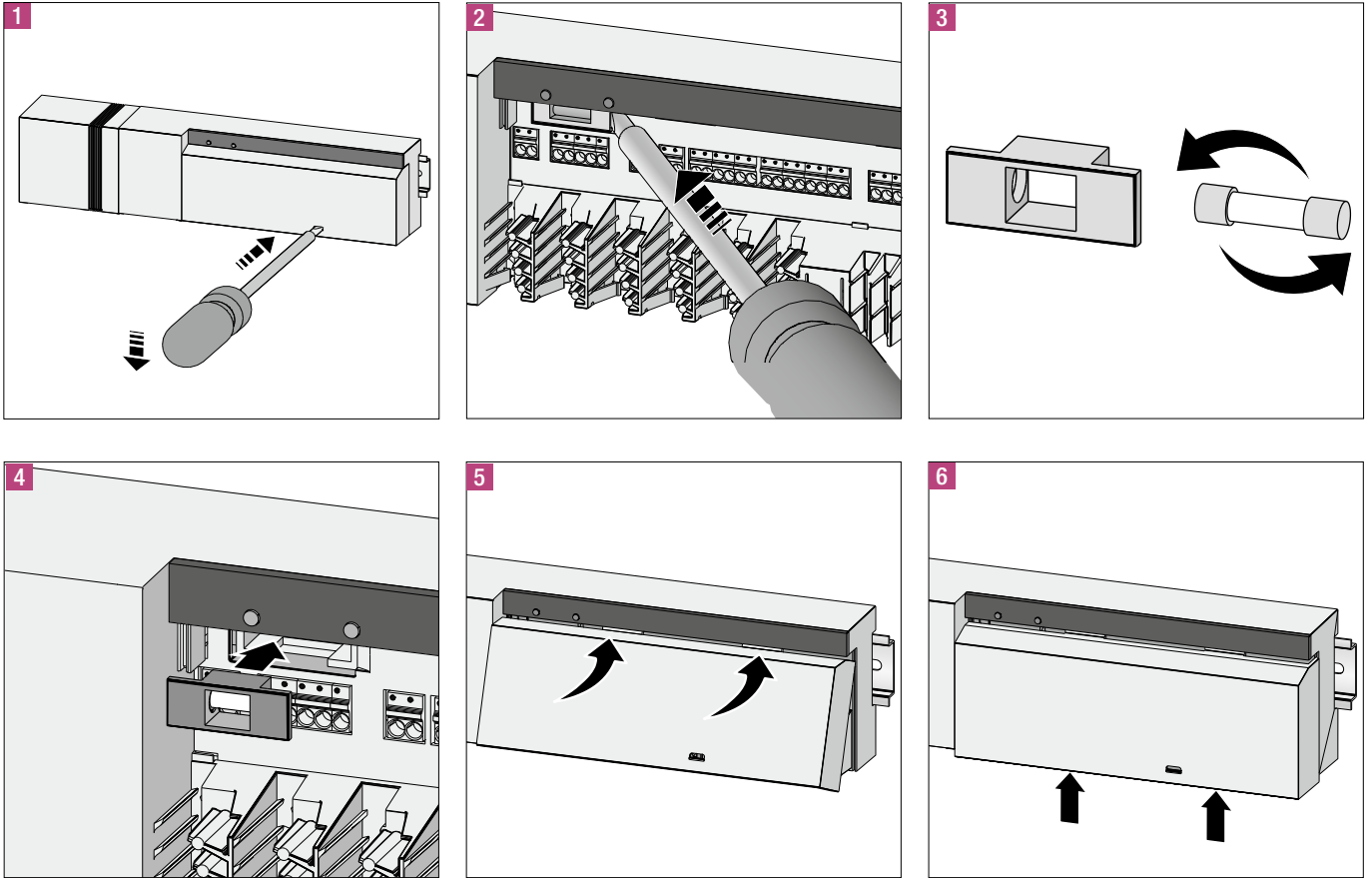
Şek. 6-2 Sigortanın deęiřtirilmesi
