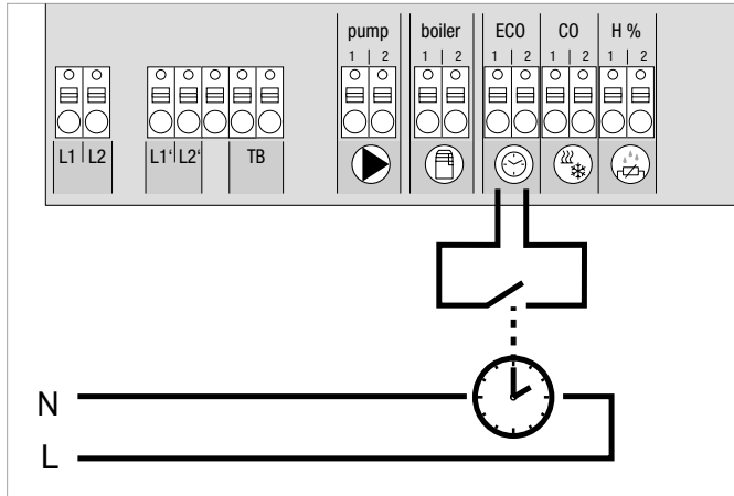
Şek. 3-7 Harici bir zamanlama modülünün bağlantısı
