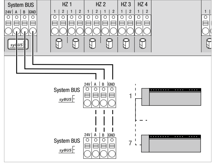
Şek. 3-9 Baz istasyonlarının Sistem BUS üzerinden bağlantısı
