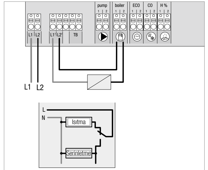
Şek. 3-6 „Boyer“ çıkışının Change Over pilot sinyali olarak kullanımı
