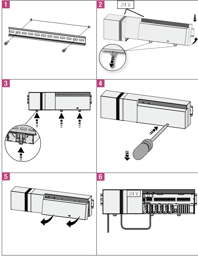
Şek. 3-1 Kurulum
