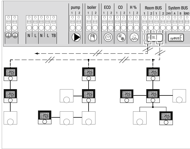
Şek. 3-8 Nea Smart oda termostatının Nea Smart Basis bağlantısı
