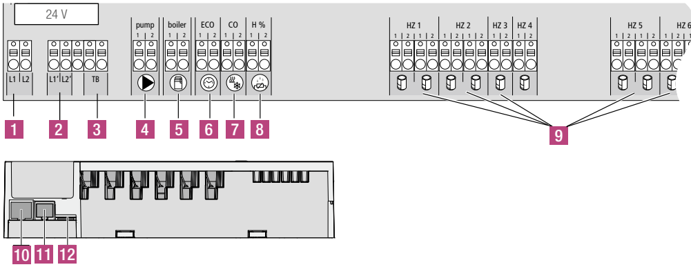
Şek. 2-3 Bağlantılar
