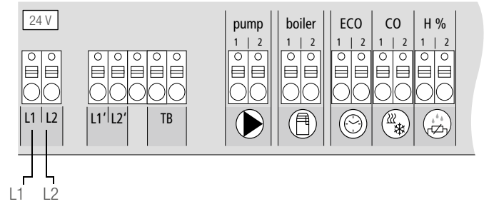
Şek. 3-2 Elektrik bağlantısı
