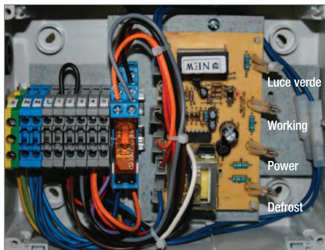
Fig. 6-1 Il quadro elettrico con la scheda elettronica
