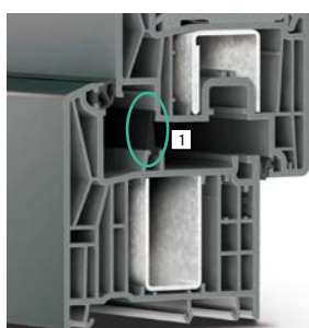
1 Middendichting
